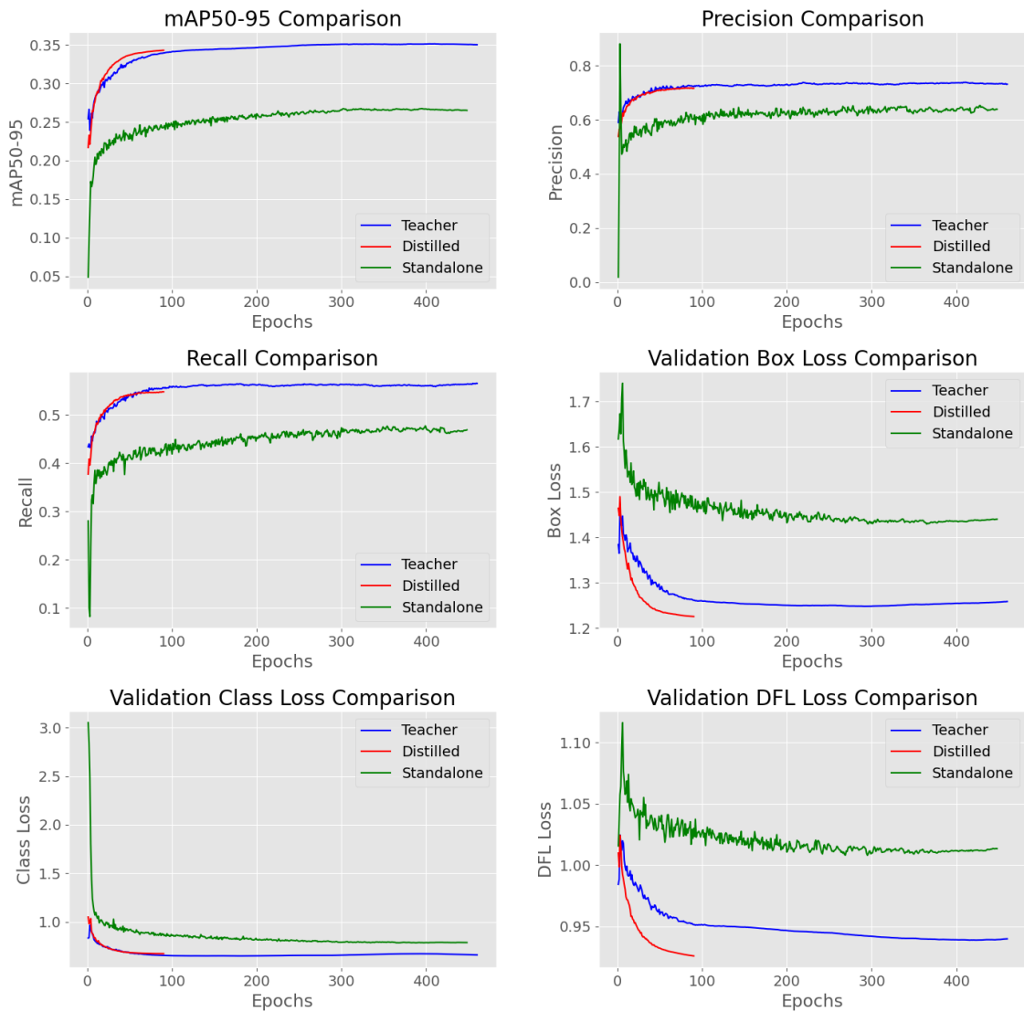
图 4.5 模型精度和损失对比
