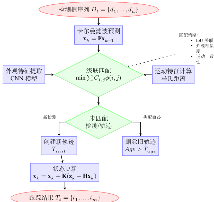
图 4.7 DeepSORT 算法框架
