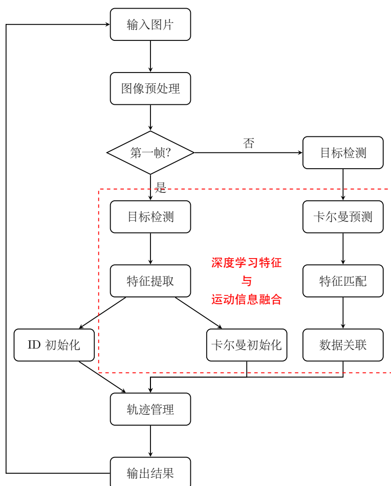
图错误!文档中没有指定样式的文字。-8 DeepSORT 跟踪框架
