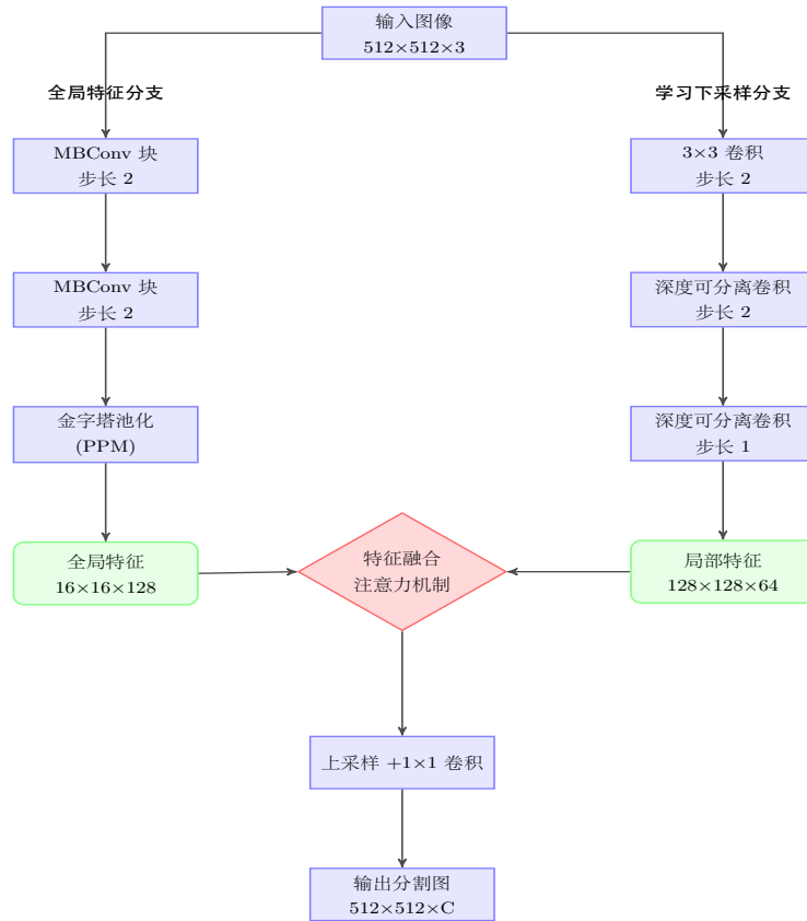
图错误!文档中没有指定样式的文字。-6 Fast-SCNN 网络架构
