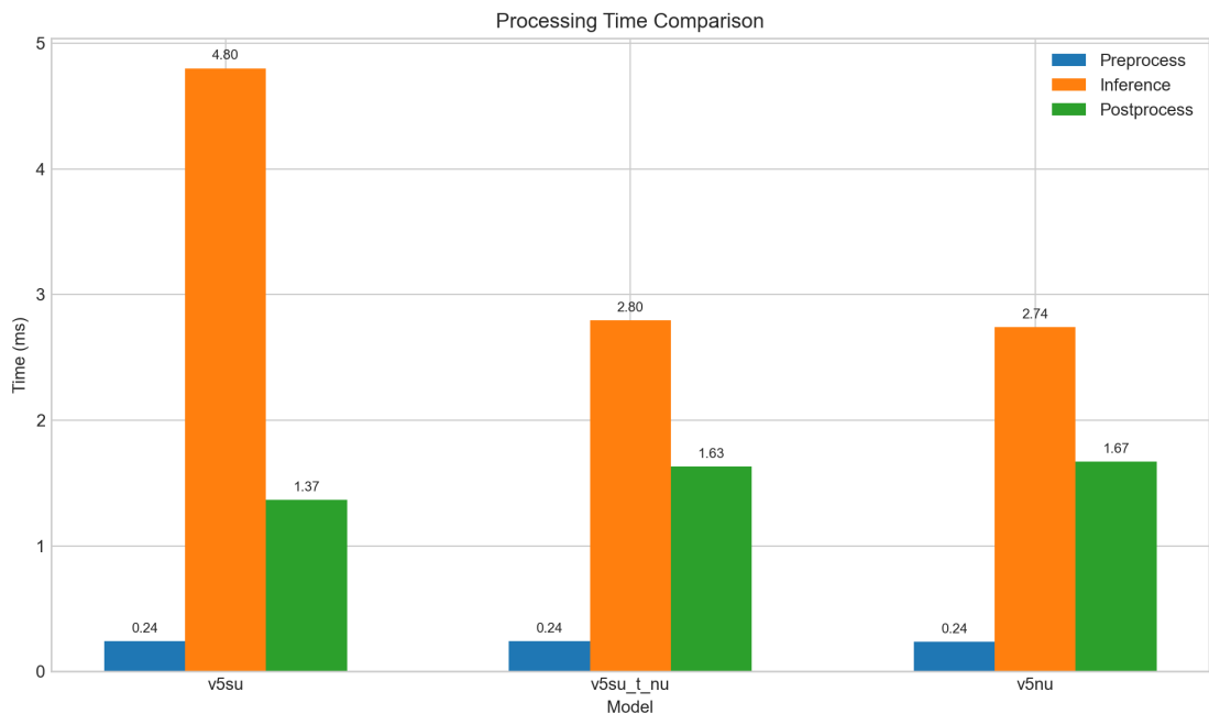
图错误!文档中没有指定样式的文字。-23 处理速度对比图
