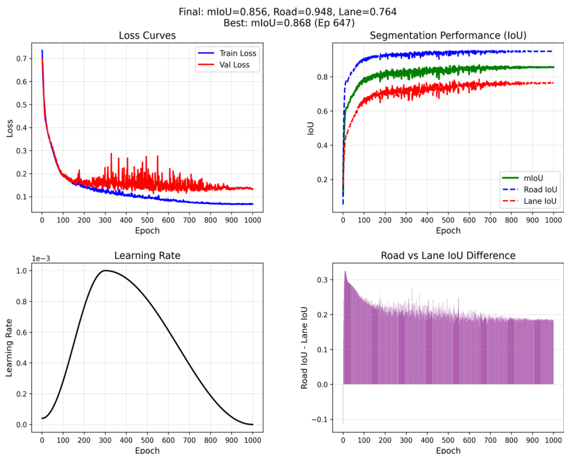
图错误!文档中没有指定样式的文字。-18 Fast-SCNN 模型训练分析
