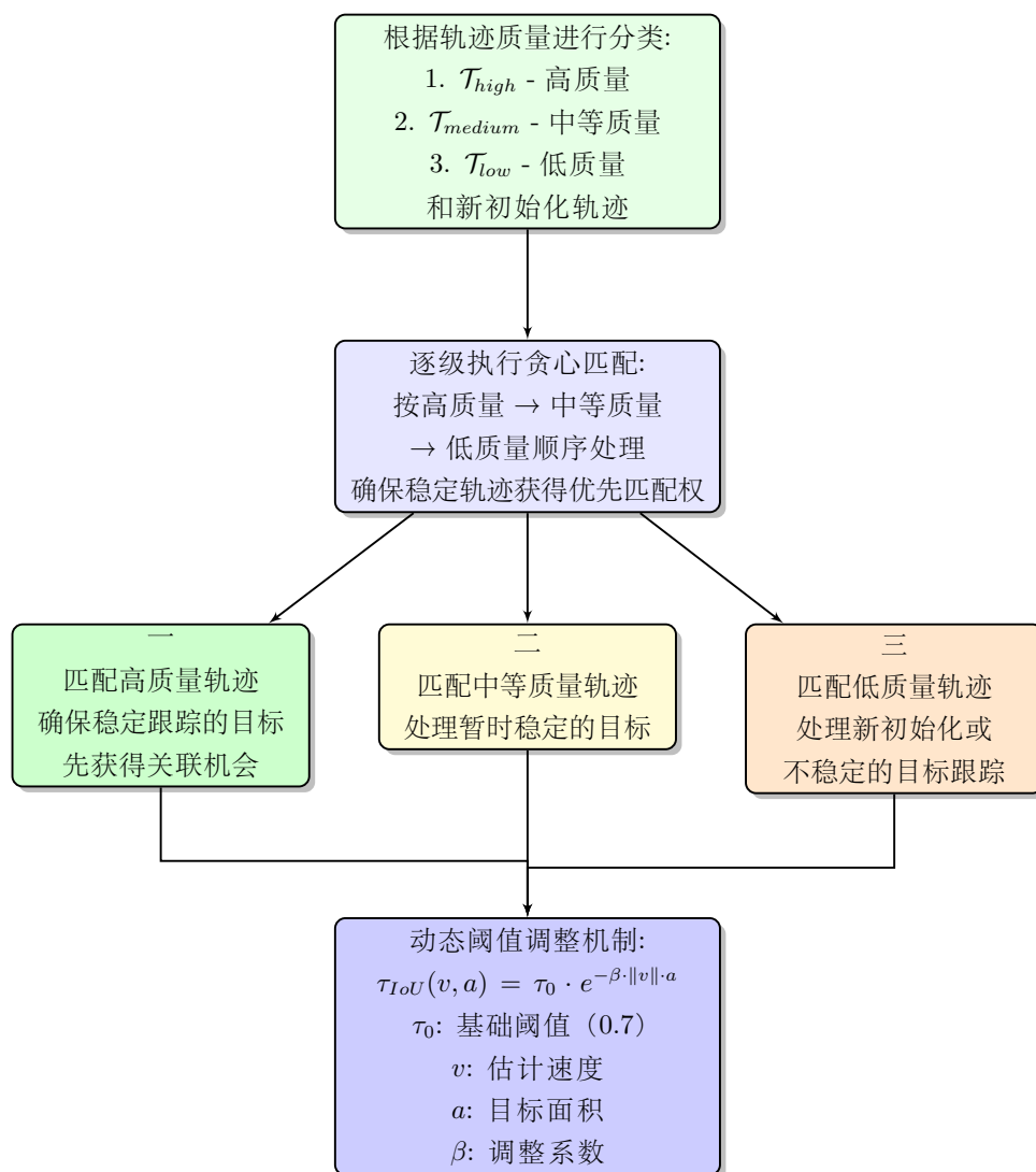
图错误!文档中没有指定样式的文字。-30 级联匹配策略
