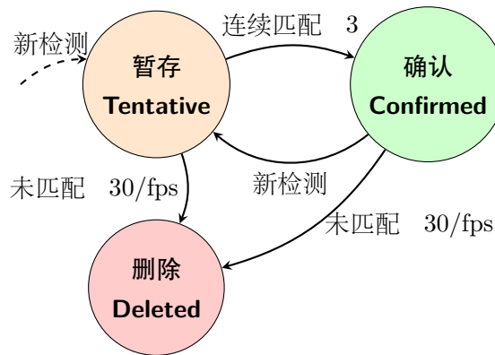
图错误!文档中没有指定样式的文字。-28 轨迹状态转换
