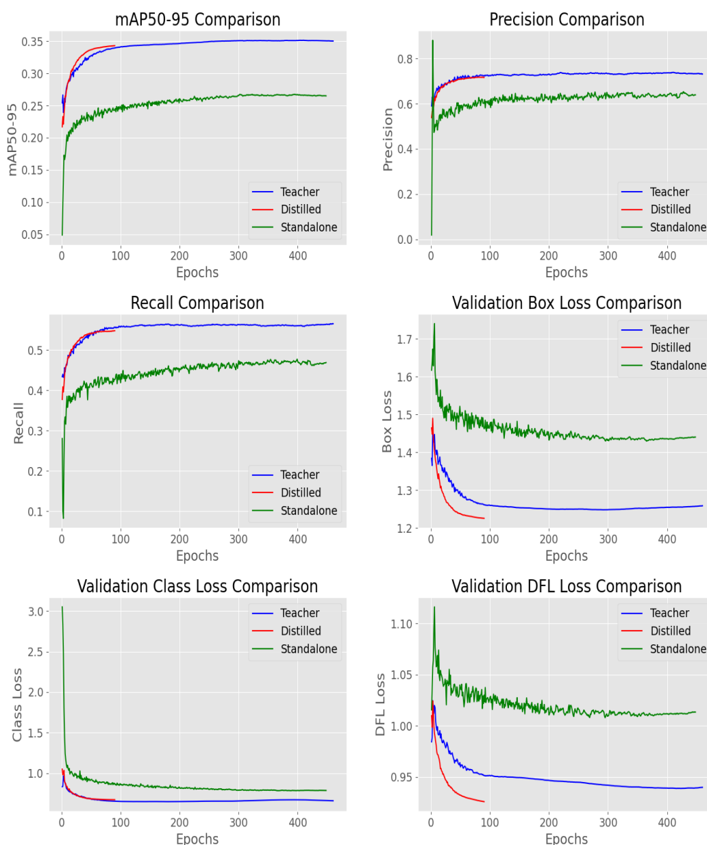
图错误!文档中没有指定样式的文字。-25 模型精度和损失对比
