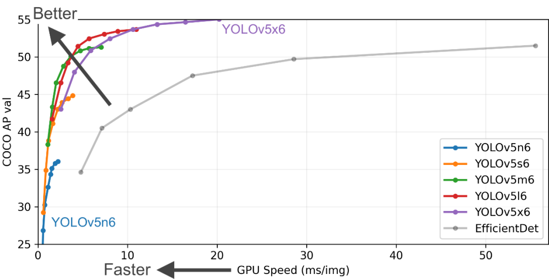
图错误!文档中没有指定样式的文字。-7 YOLOv5 模型在 COCO 数据集上测试结果 各个尺度的预训练参数如表 1 所示 [37] 。
