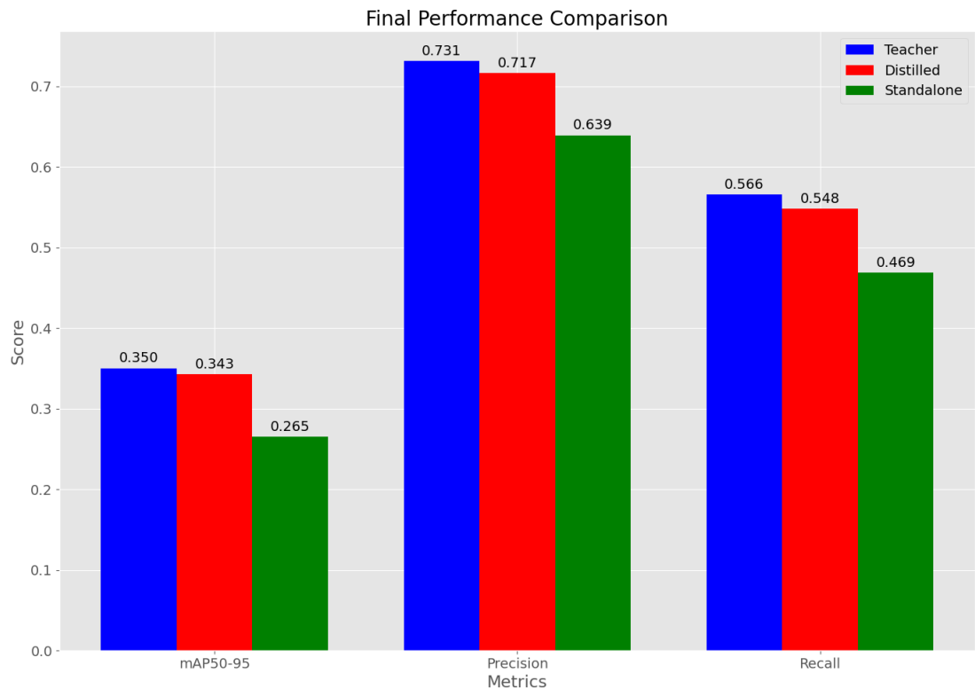
图错误!文档中没有指定样式的文字。-26 模型综合性能比较
