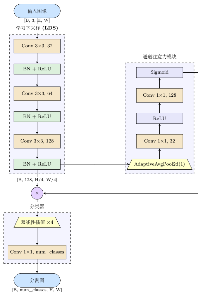
图错误!文档中没有指定样式的文字。-17 改进的网络结构
