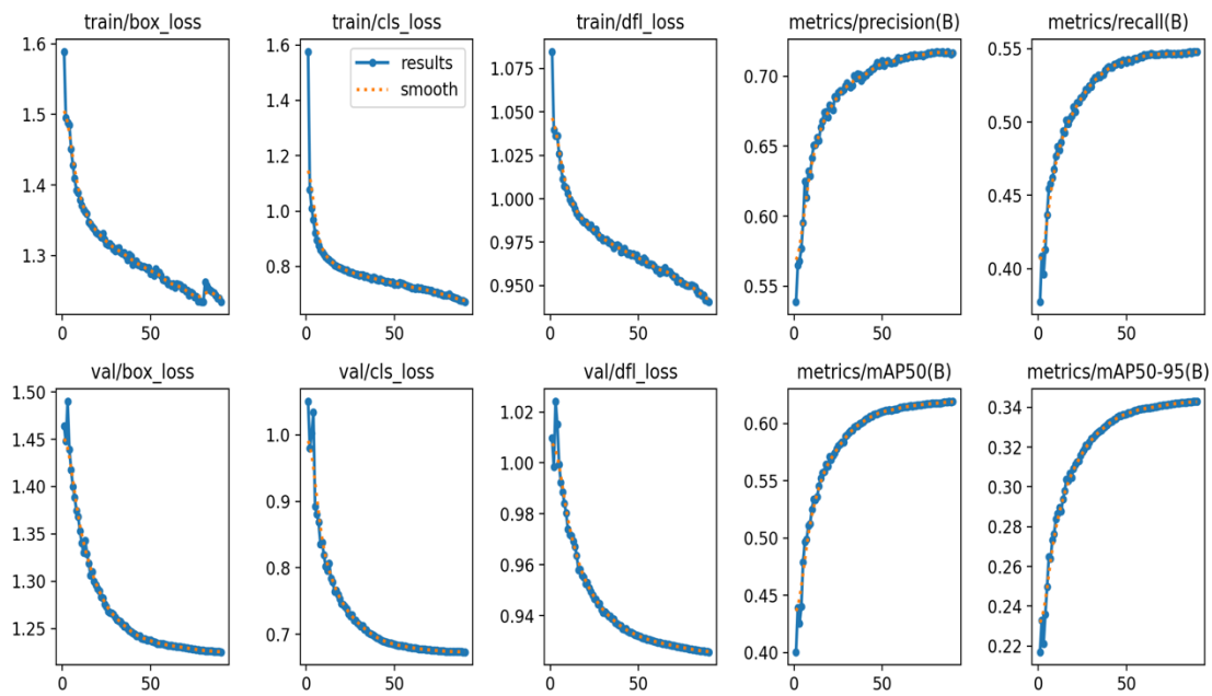
图错误!文档中没有指定样式的文字。-21 模型训练验证性能曲线
