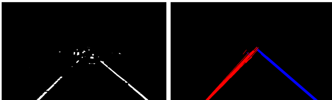
图错误!文档中没有指定样式的文字。-14 霍夫变换直线检测效果
