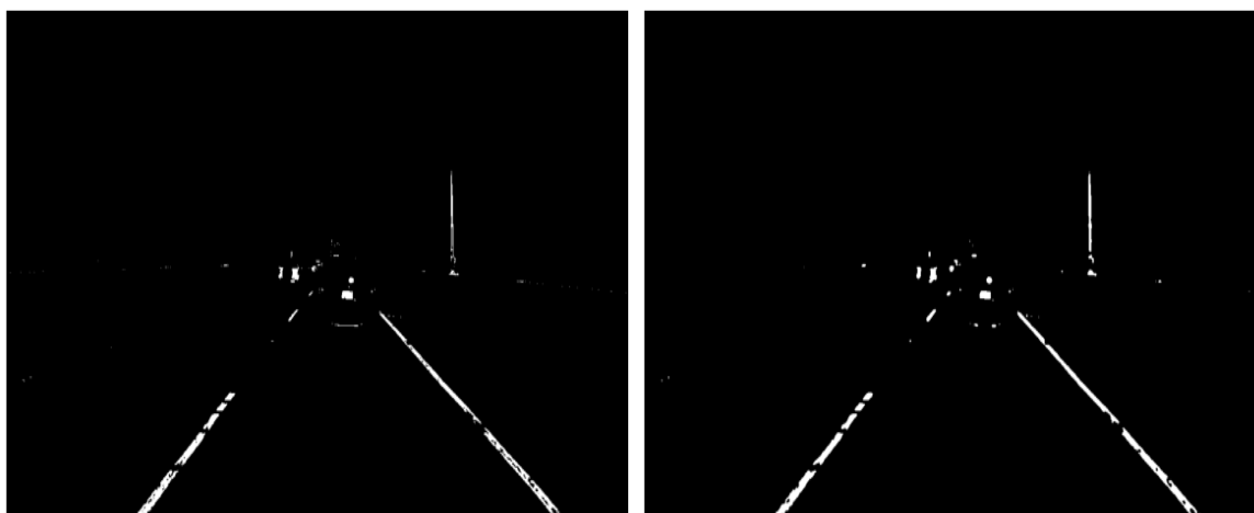
图错误!文档中没有指定样式的文字。-10 多尺度 DoG 边缘检测效果
