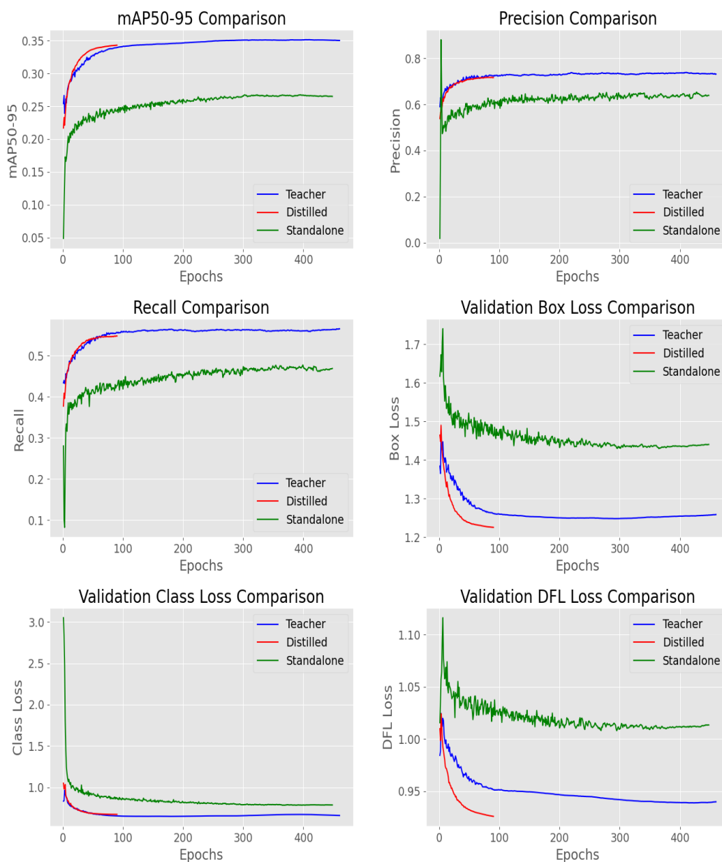
图 4-6 模型精度和损失对比
