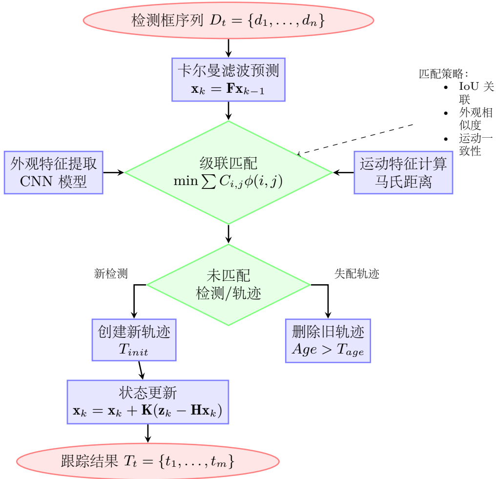
图 4-8 DeepSORT 算法框架
