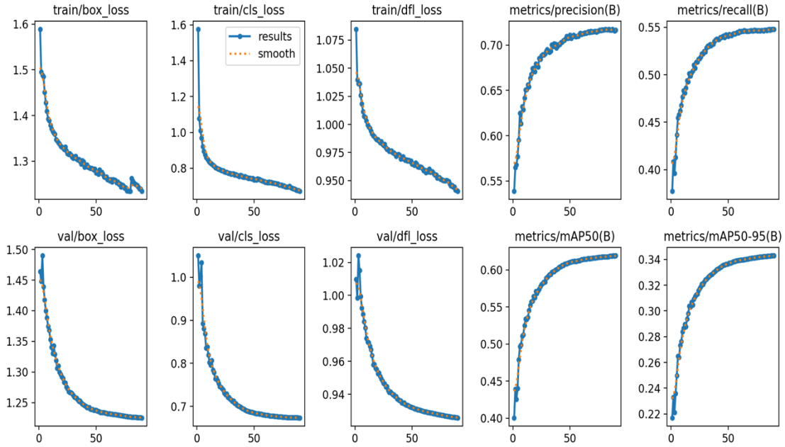
图 4-2 模型训练验证性能曲线
