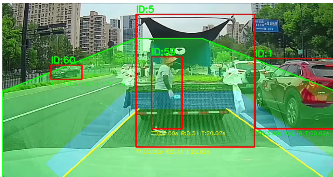
(b) 第 300 帧跟踪结果
