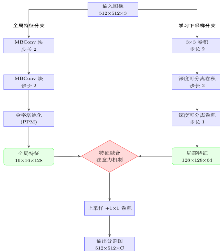
图 2-5 FastSCNN 网络架构
