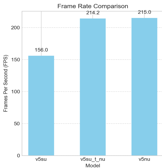
图 4-5 帧率对比图
