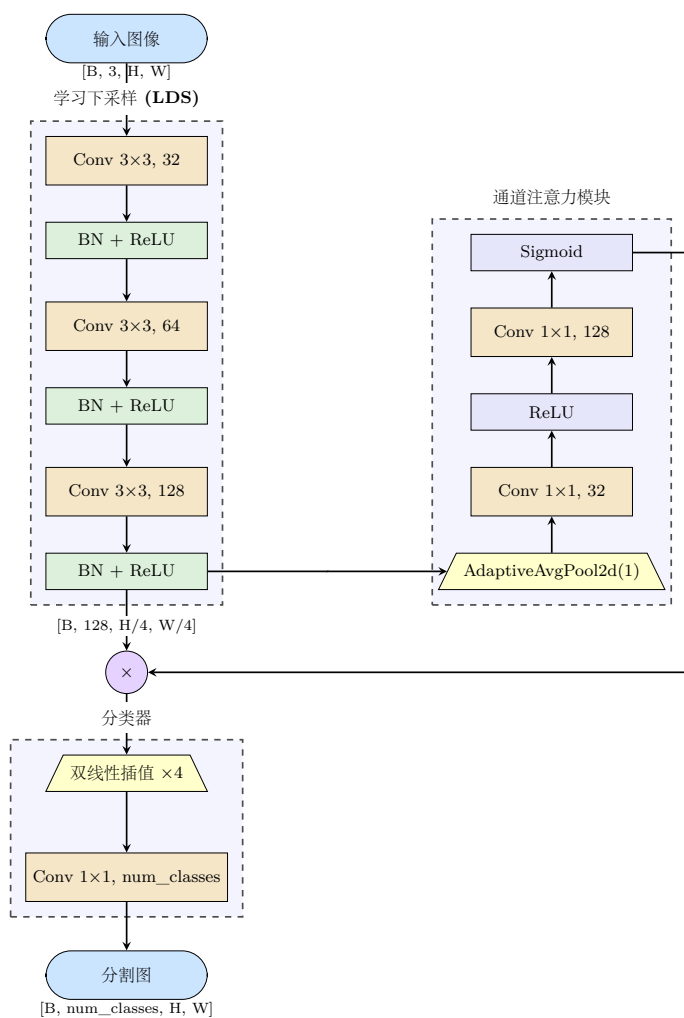
图 3-9 改进的网络结构
