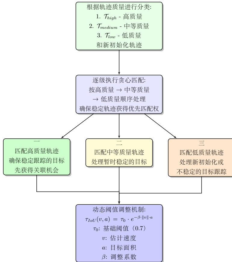
图 4-11 级联匹配策略
