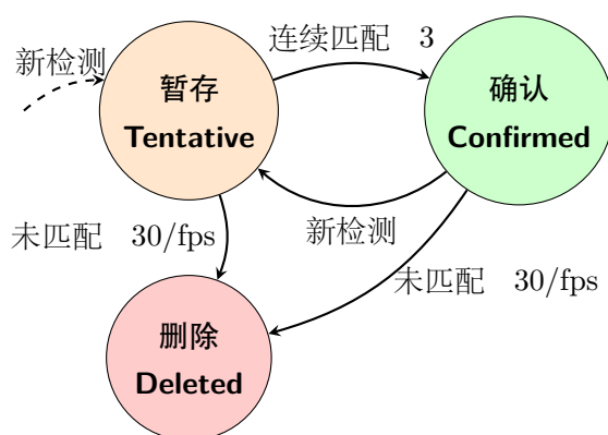
图 4-9 轨迹状态转换
