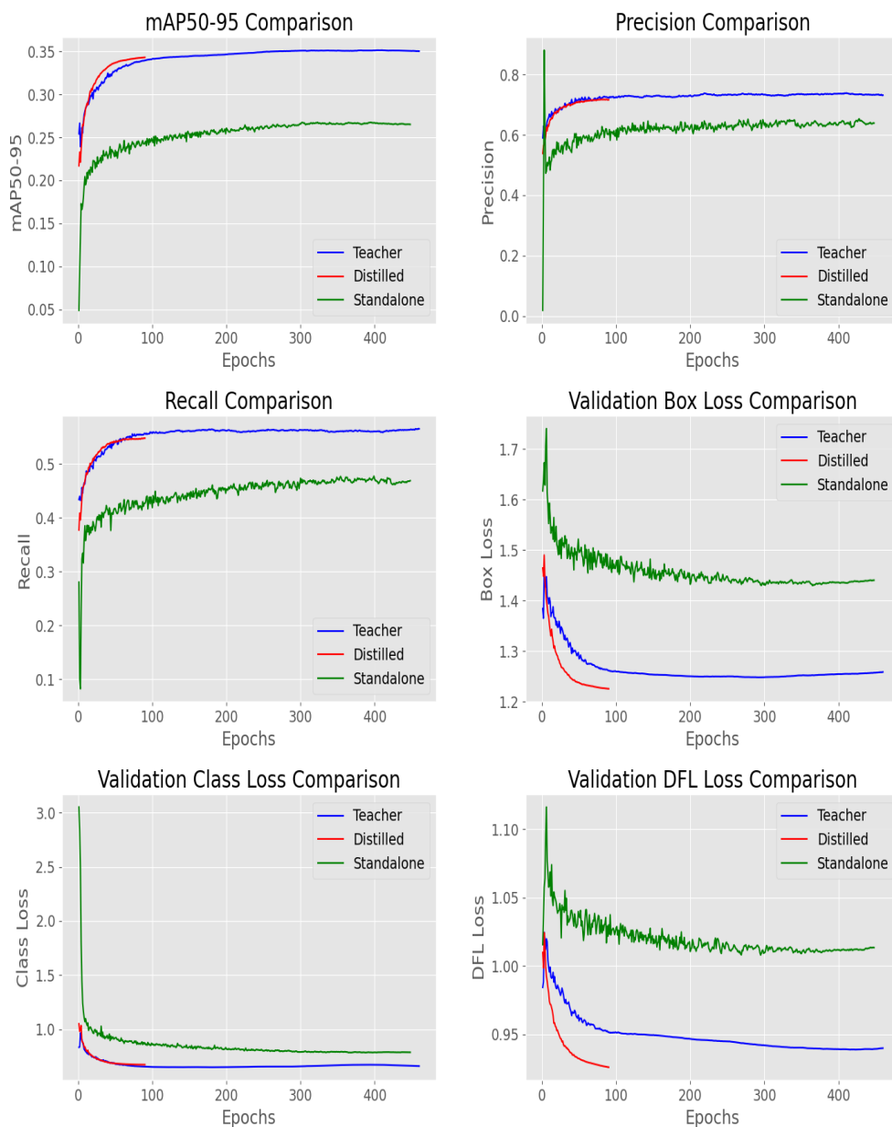
图 4-6 模型精度和损失对比
