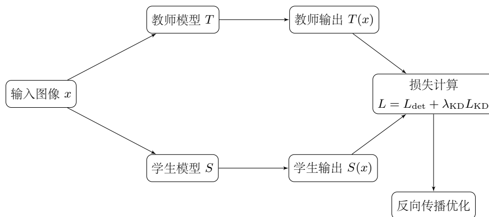
图 4-3 知识蒸馏训练流程
