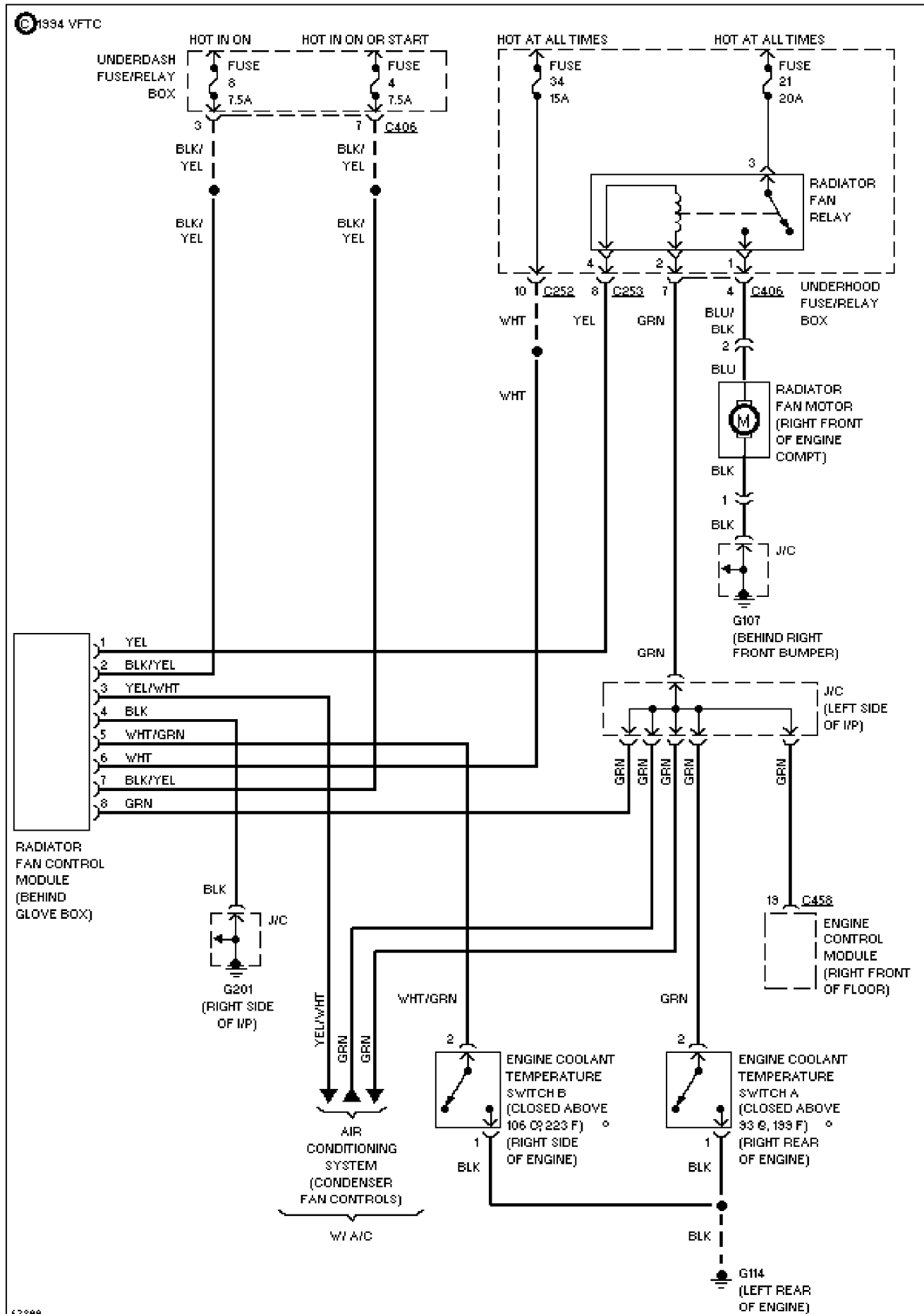
Cooling Fan Circuit
