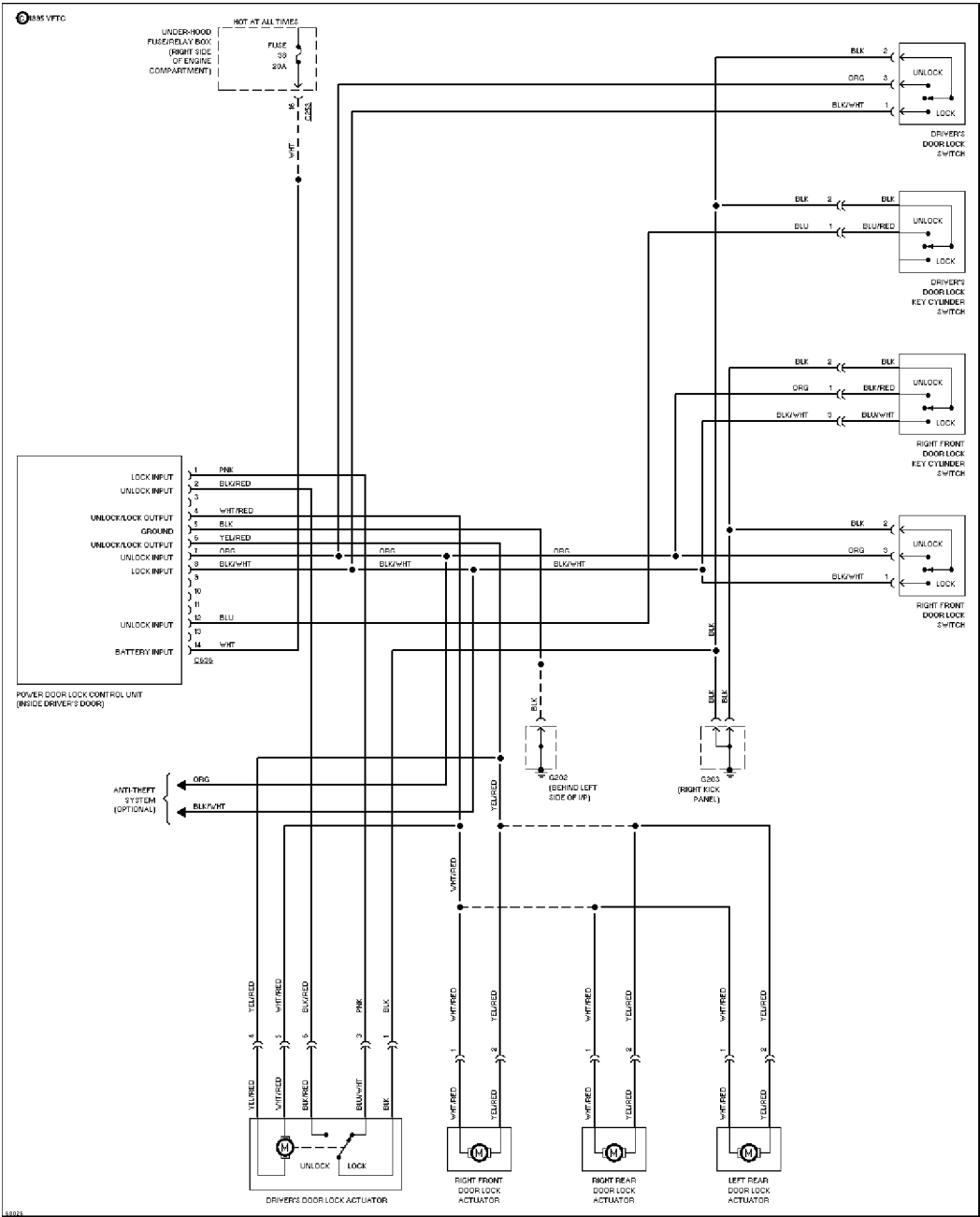
Power Door Lock Circuit, Coupe & Sedan
