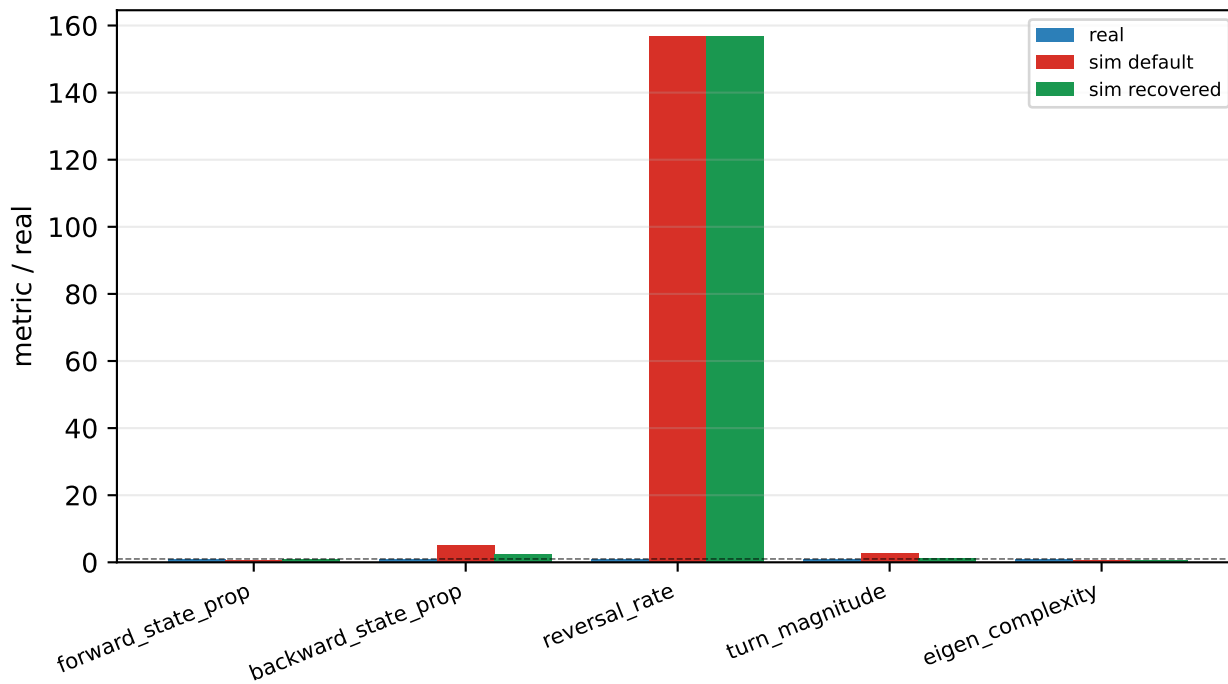
BAAIWorm (Zhao 2024) — OWMD-N2 reference
