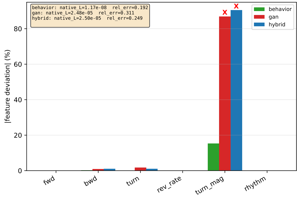
modWorm 50d (CMA-ES sep, pop16, 30 iter, scale=0.10)
