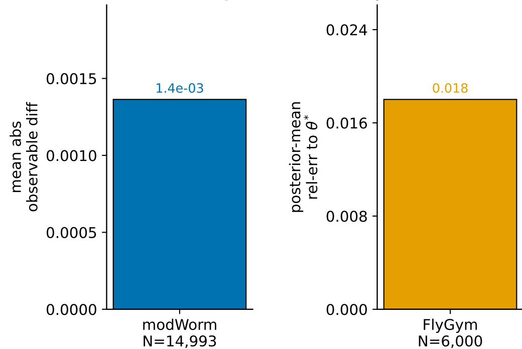
A Amortized posterior recovery (NPE-MAF)
