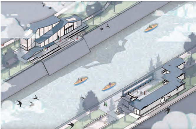
■ SITE B
