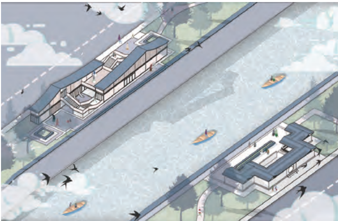
■ SITE C
