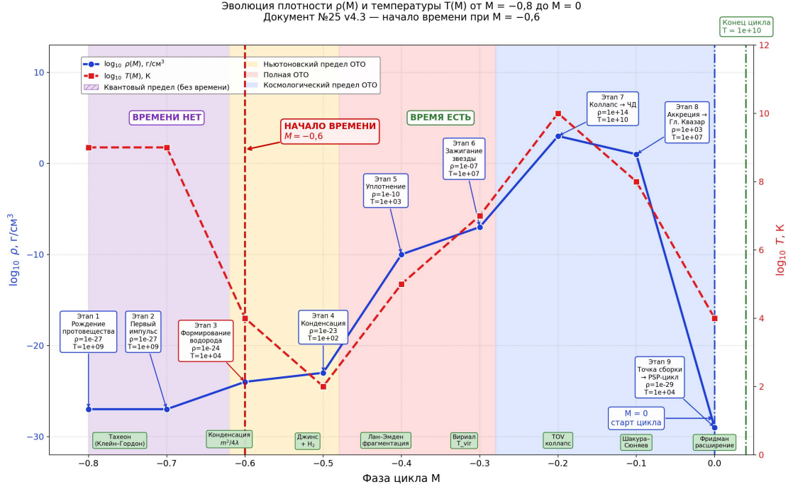
Рисунок 1: Эволюция плотности \rho(M) (синяя кривая) и температуры T(M) (красная пунктирная) в модели PSP. Вертикальная линия при M = -0,6 отмечает начало времени.
