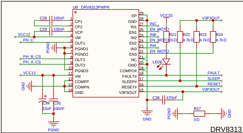
DRV8313
