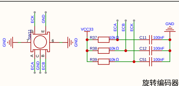
旋转编码器
