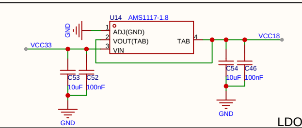
LDO
