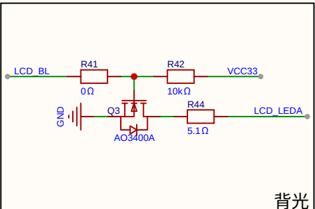
背光
