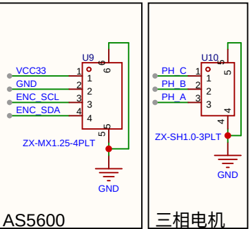
AS5600
