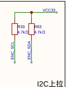
I2C上拉
