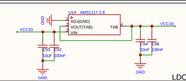
LDO
