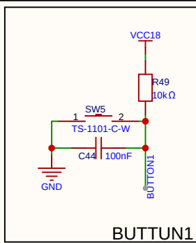
BUTTUN1
