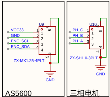
AS5600
