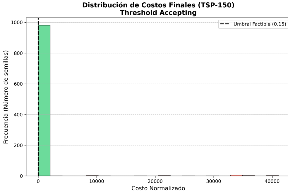
Figura 1: Distribución de los costos finales sobre 1,000 ejecuciones (semillas) de la 0 a la 1000 para la instancia TSP-150. El umbral objetivo de 0.15 está marcado en línea punteada.
