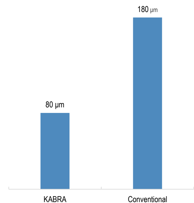
【SiC ingot material loss】
