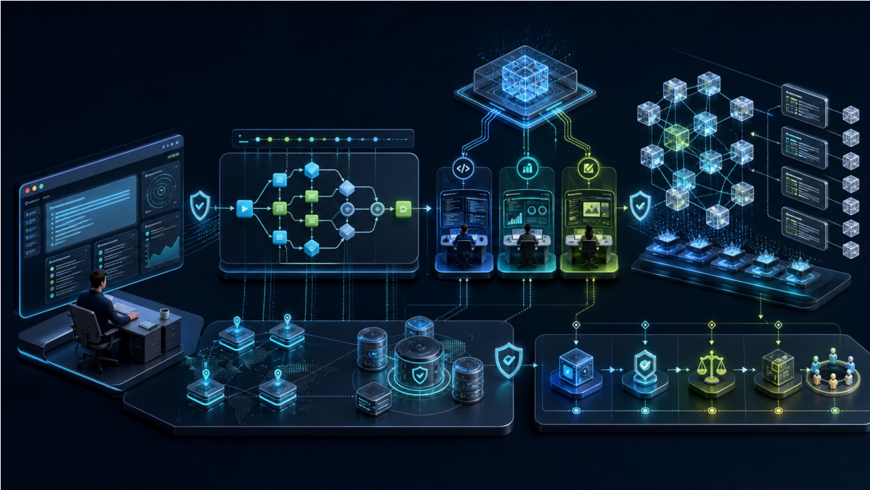
图 1：复杂目标 → DAG 编译 → 多 Agent 执行 → 复核验收 → PinMe/IPFS 成果 → 结算治理
