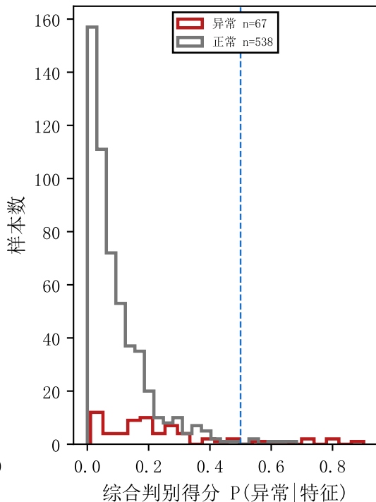
判别得分分布（异常 67/605，类不平衡）
