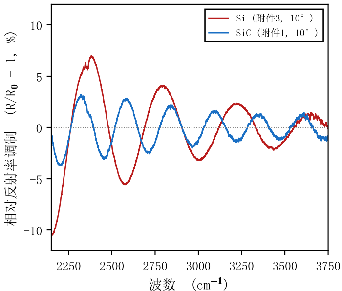
相对调制深度 (Si vs SiC)
