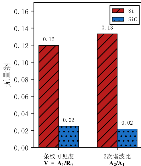
可见度 / 2次谐波比
