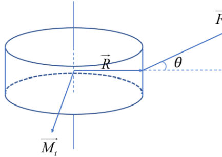
图11 单个力对圆柱产生的力矩
