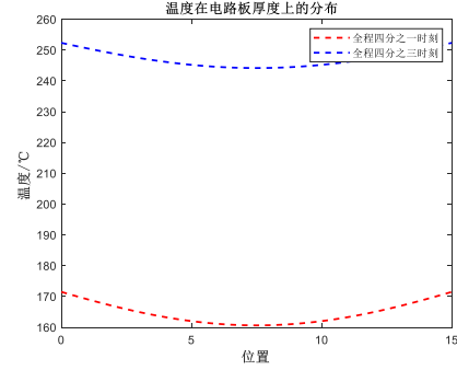
图 9 温度在电路板厚度上的分布
