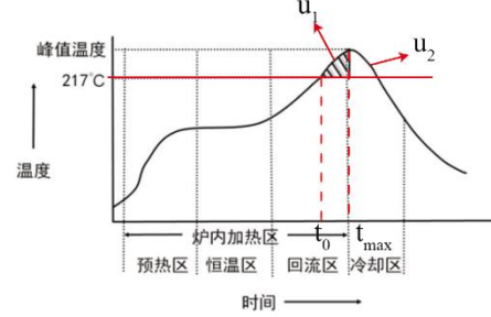
图 18 炉温曲线图
