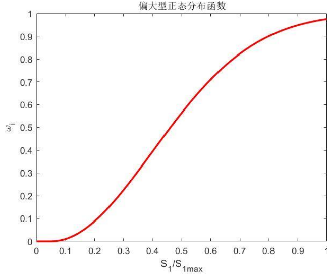
图 19 偏大型正态分布
