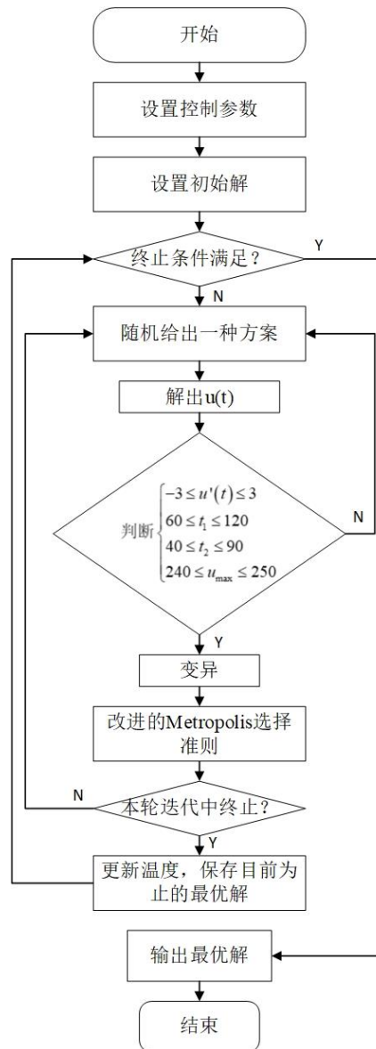
图 14 模拟退火算法的流程示意图
