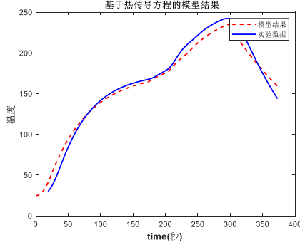
图 8 基于热传导模型结果
