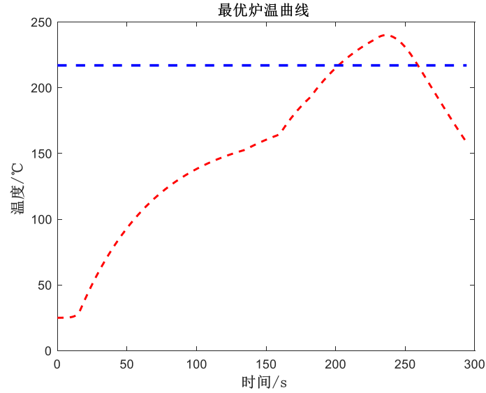
图 21 最优解下的炉温曲线
