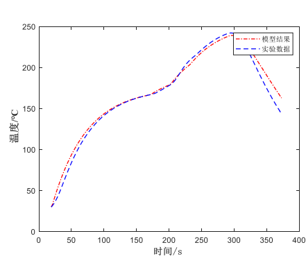
图 24 k 值取定值时模型结果
