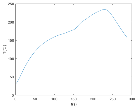
图 20: 问题四炉温曲线
