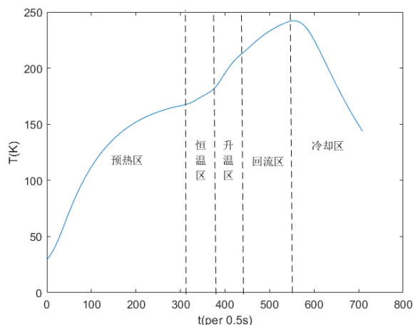
图 2: 实际炉温曲线
