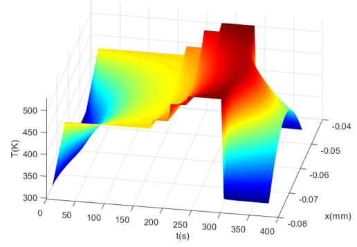
图 9: 工件整体温度分布
