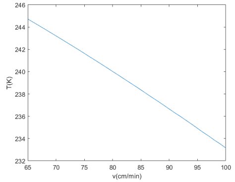
图 15: 峰值温度随过炉速度变化曲线
