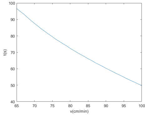
图 14: 温度大于 217^{\circ}\text{C} 时间随速度变化曲线
