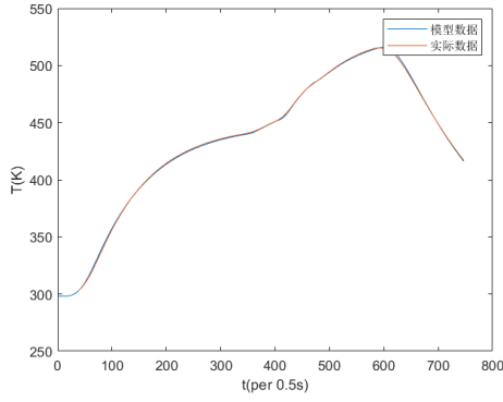
图 8: 实验炉温曲线对比
