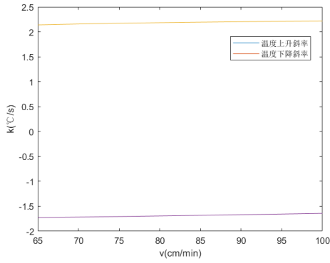
图 12: 温度升降斜率与速度关系
