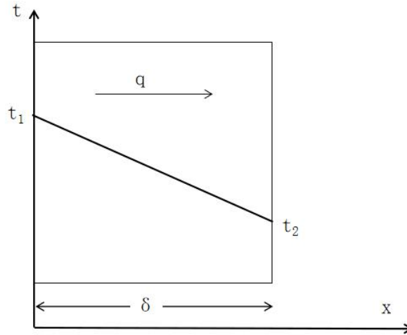
图 2、平板稳态导热示意图
