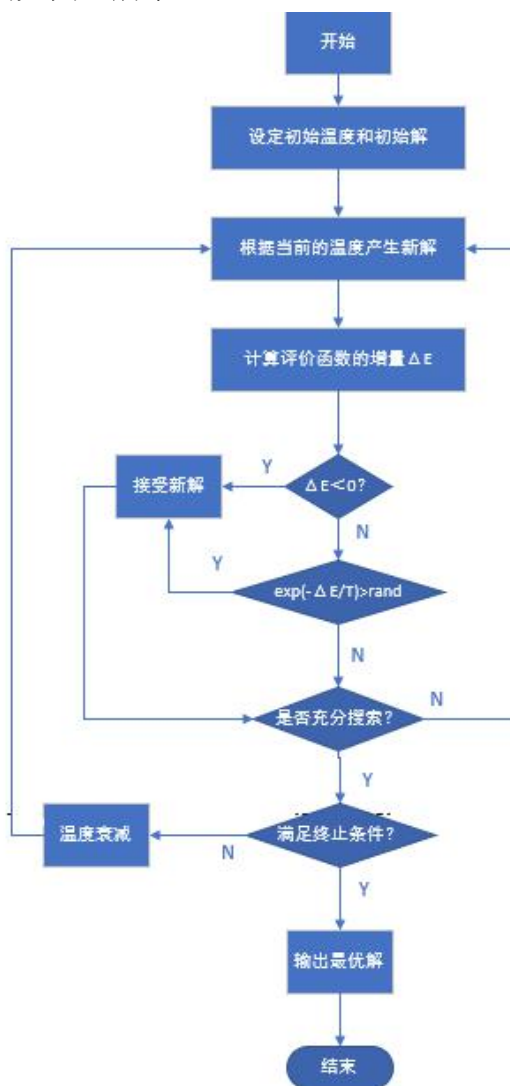
图 8、模拟退火算法流程图
