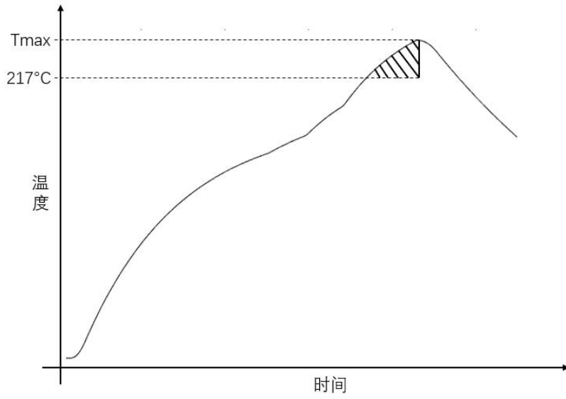
图 7、峰值温度覆盖面积示意图
