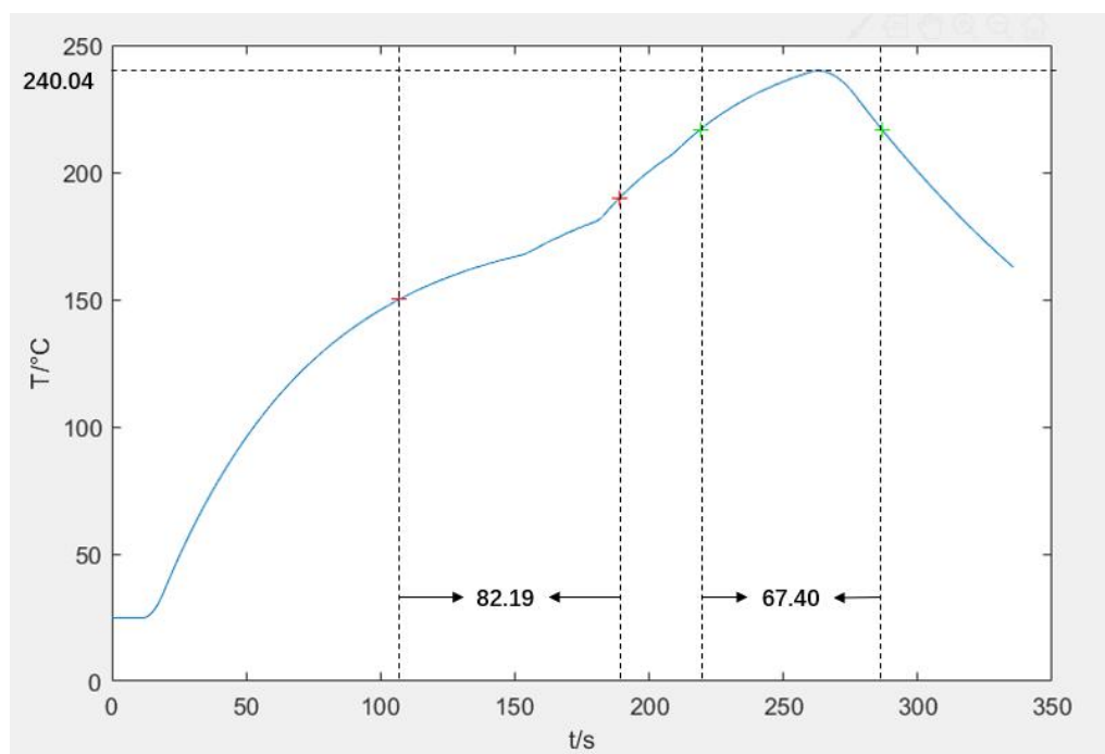
图 6、过炉速度=77.85cm/min 时的炉温曲线
