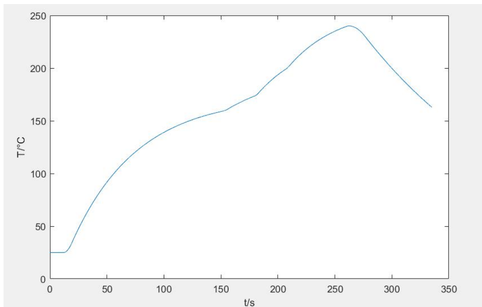
图 5、第一问条件下的炉温曲线
