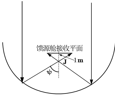
图 11 理想抛物面焦点位于接收平面以下
