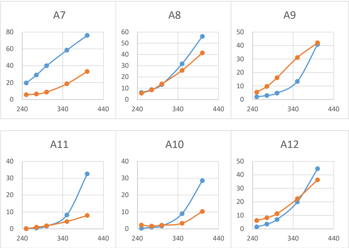
图 12: 催化剂组合 A7-A12 下相关性图 (%)
