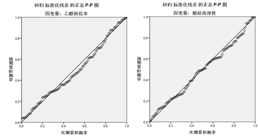
图 7：回归标准化残差的正态 P-P 图
