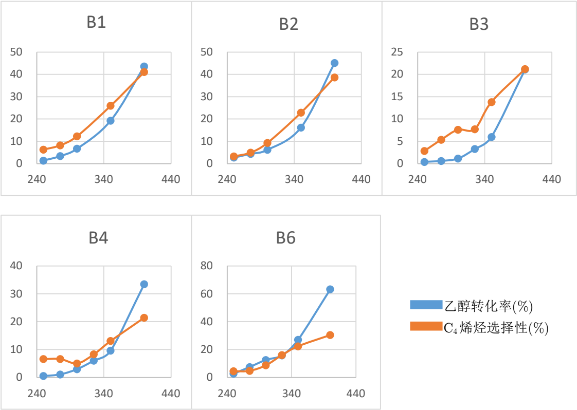
图 14：催化剂组合 B1-B4、B6 下相关性图
