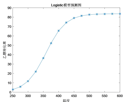
图 2 B1 组的乙醇转化率趋势预测图
