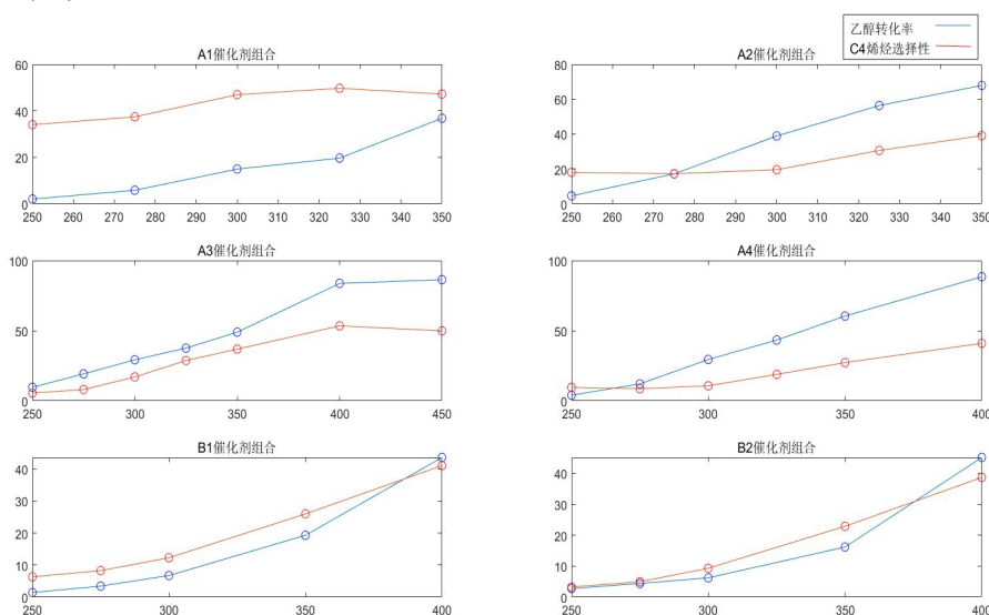
图 1 乙醇转化率和 C4 烯烃选择性随温度变化散点图(部分)
