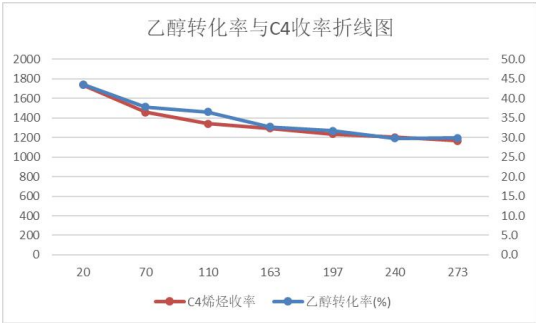
图 6 乙醇转化率与 C4 收率折线图
