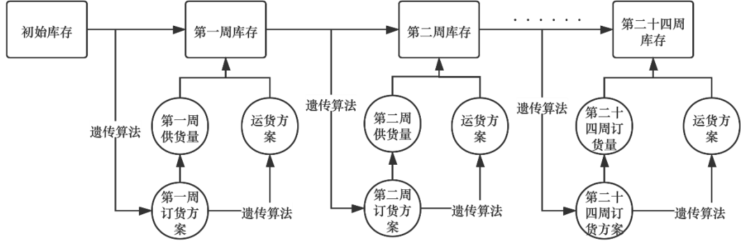
图 2：问题二的多目标规划模型
