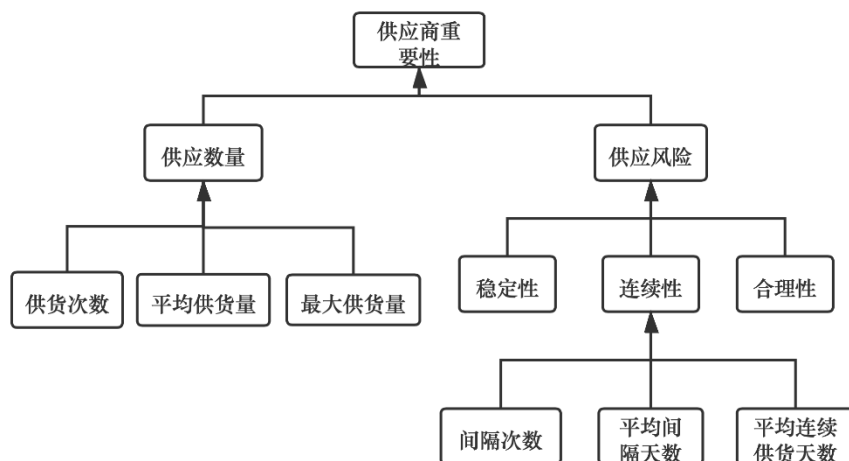
图 1：问题一多指标评价模型
