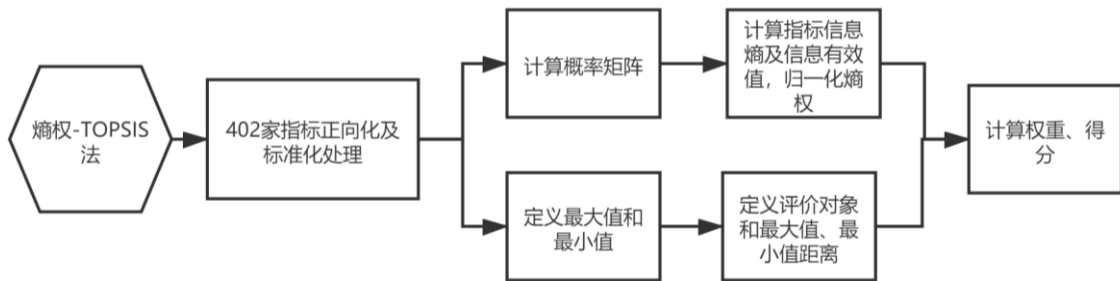
图 8：熵权-TOPSIS 法流程图
