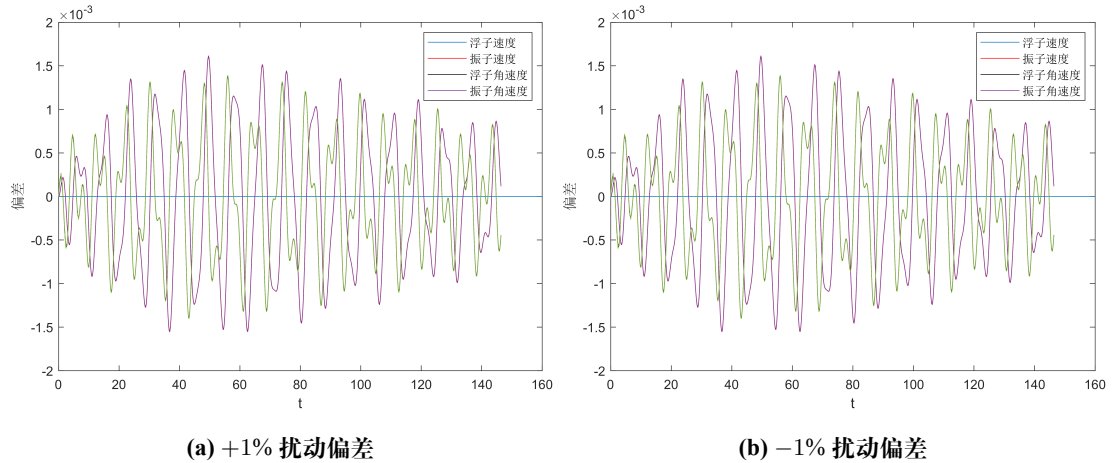
图 14 运动过程中 \pm 1\% 扰动偏差
