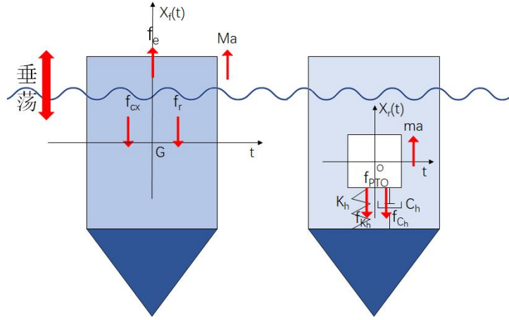
图2 垂荡运动受力分析示意图
