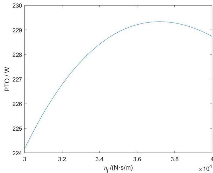
图 4 PTO 关于 \eta_i 的函数图 2
