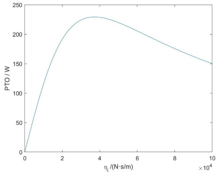
图 3 PTO 关于 \eta_i 的函数图 1
