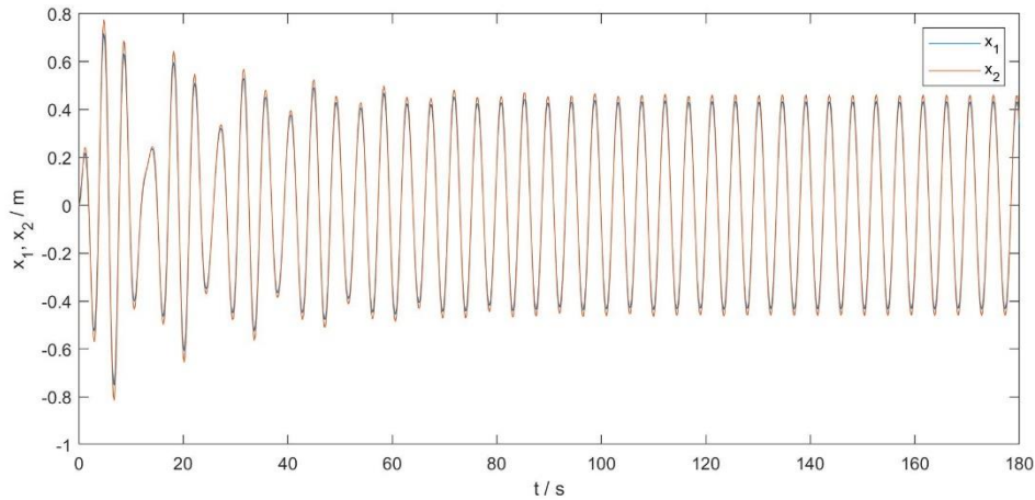
图 1 浮子与振子位移 x_1 、 x_2 随时间 t 的变化曲线
