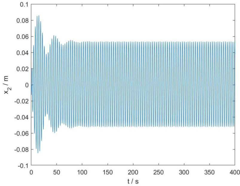
图 8 x_2 关于时间的变化
