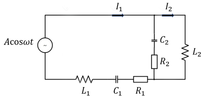
图 6 力电比拟等效电路图
