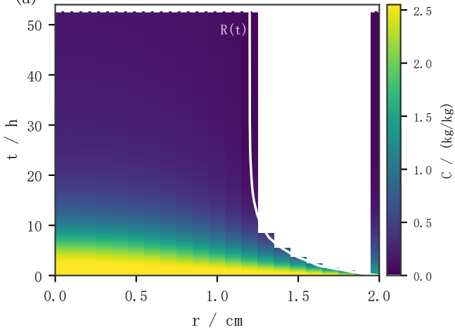
(a) Q4 收缩域含水率场 (物理坐标, 域外留空)
