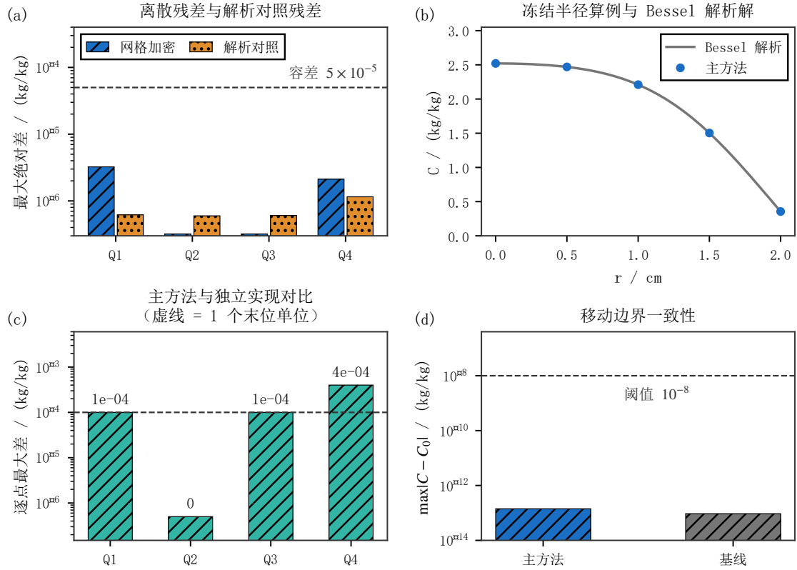
图 9 数值可信度的四类证据。(a) 网格加密残差与解析解对照残差；(b) 问题四的冻结半径算例与 Bessel 级数解析解的对照；(c) 主方法与独立实现的逐点最大差，虚线为一个末位单位对应的容差；(d) 问题四关闭表面传质后干基含水率的偏移量与其阈值。
