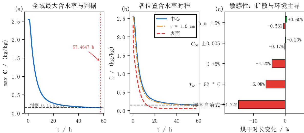
图 5 长时程烘干过程与敏感性。(a) 全域最大干基含水率随时间的演化与 0.15 kg/kg 判据；在题目给定的 h_m 、附录 3 经验式与恒温段环境口径下，判据于 57.4647 h 首次越过。(b) 三个位置的含水率时程。(c) 单项扰动对烘干时长的影响。
