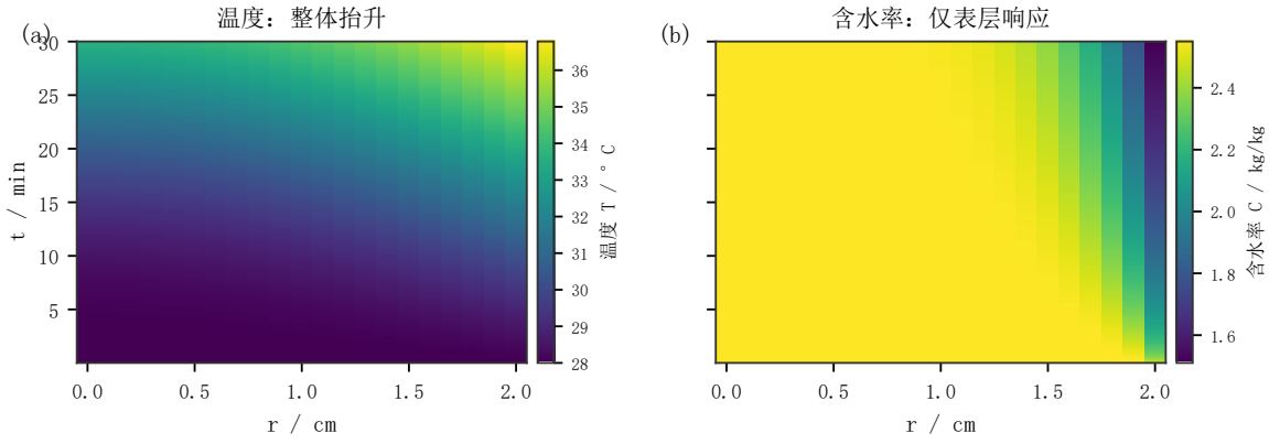
图 4 预热阶段温湿场的完整时空分布（附录图）。左：温度；右：干基含水率。
