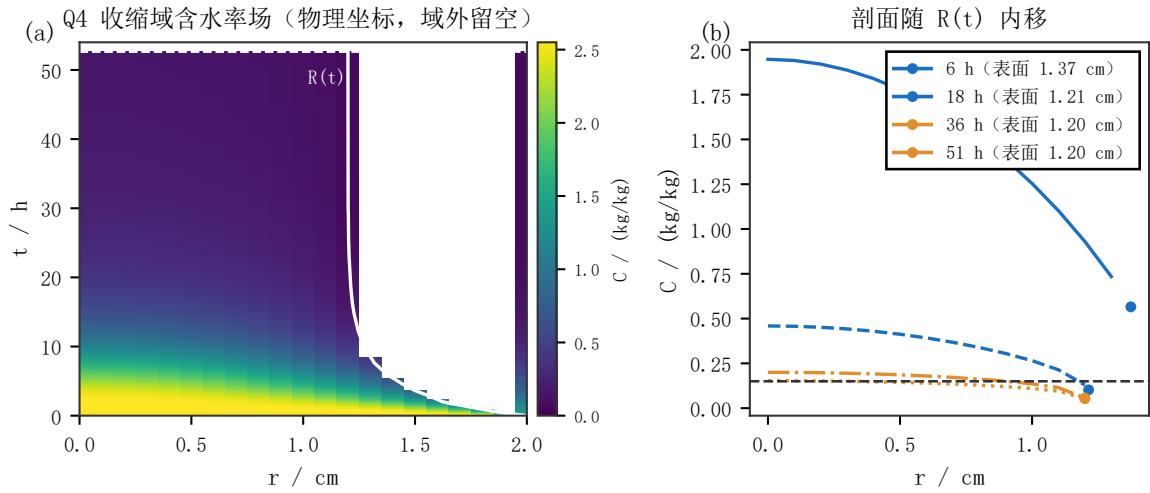
图 8 问题四收缩域内的含水率场 (附录图, 物理坐标)。(a) 径向-时间分布, 白线为 R(t) , 域外留空; (b) 四个时刻的径向剖面, 圆点为该时刻的表面位置。
