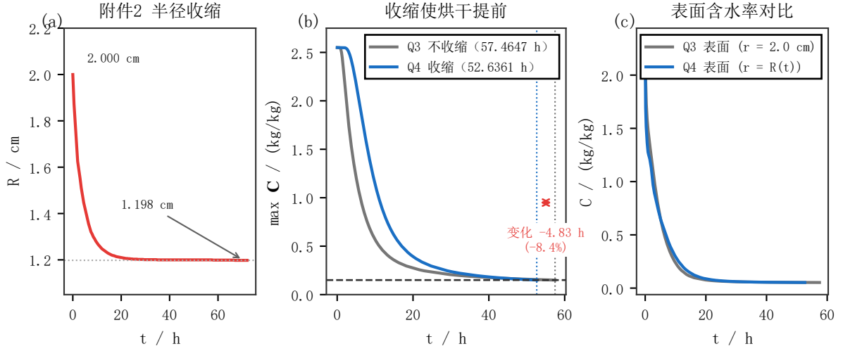
图 7 尺寸收缩对烘干时长的影响。(a) 半径按附件 2 由 2.000 cm 收缩到 1.2 cm (40.1%)。(b) 同判据线下, 考虑收缩 (52.6361 h) 比不考虑收缩 (57.4647 h) 提前 -4.8286 h。(c) 表面含水率对比。
