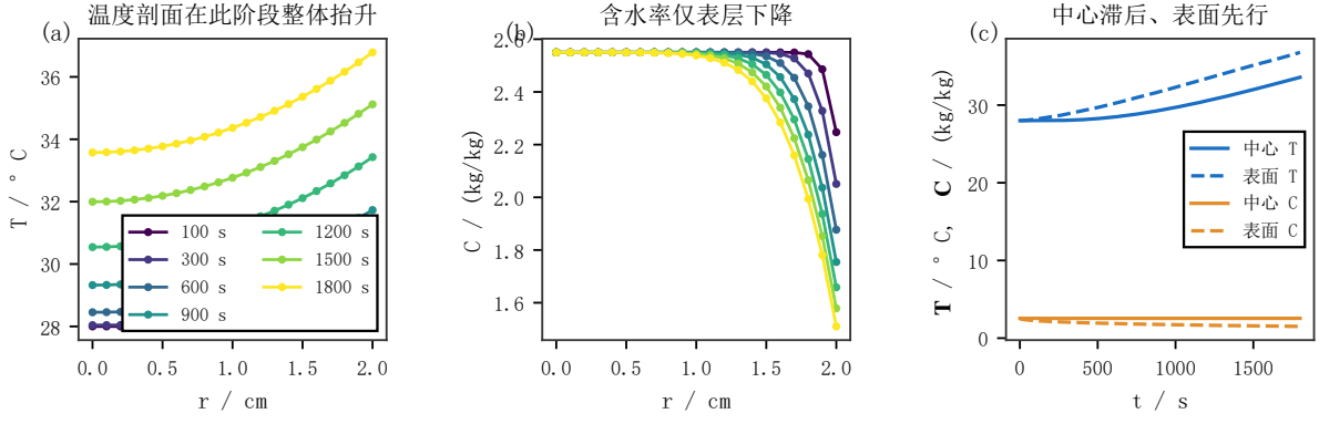
图 3 预热平衡阶段 (0 ~ 1800 s) 的温度与水分场。(a)、(b) 为七个报告时刻的径向剖面；(c) 为中心与表面时程。在题目给定的 h_m 与附录 2 经验式下，1800 s 时中心温度 33.5753^{\circ}\text{C} 、表面 36.7856^{\circ}\text{C} ；干基含水率中心仍为 2.55\text{ kg/kg} ，仅表面降至 1.5102\text{ kg/kg} 。
