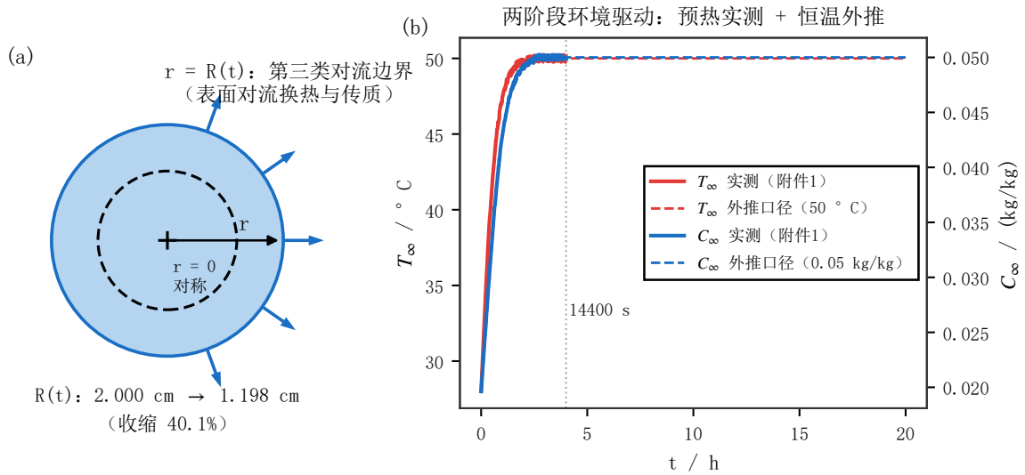
图 2 模型几何与边界驱动。(a) 药材按一维径向轴对称处理， r = 0 处对称、 r = R(t) 处第三类对流；(b) 预热阶段的环境温湿度取附件 1 实测序列（线性插值），14400 s 之后按已确认口径维持 T_\infty = 50 \text{ }^\circ\text{C} 、 C_\infty = 0.05 \text{ kg/kg} 。该外推为 建模口径 ，并非实测数据。
