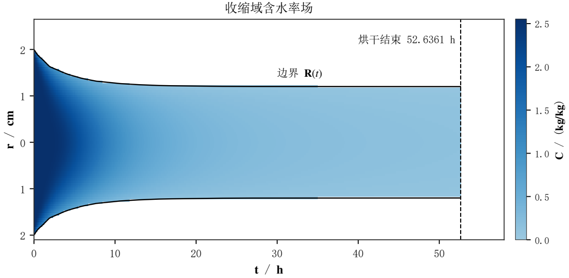
图 11 问题四收缩域含水率场（附录图）
