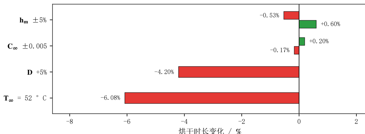
图 9 烘干时长对单项扰动的响应（问题二与问题三）
