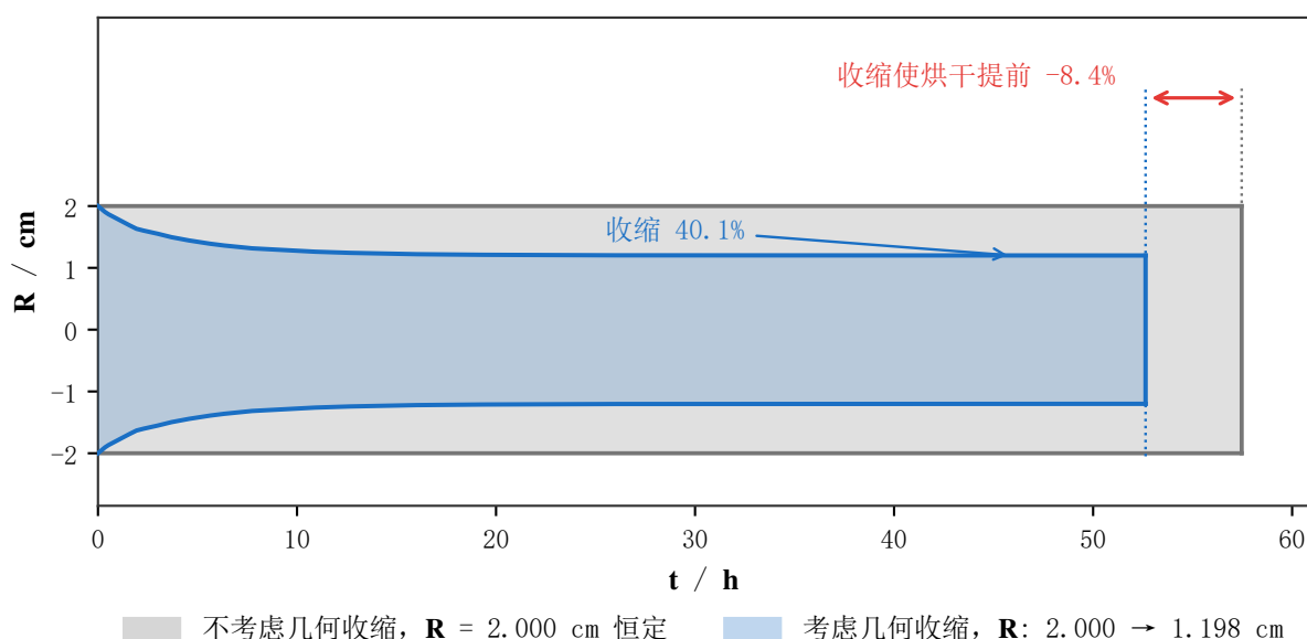
图 10 尺寸收缩对烘干时长的影响
