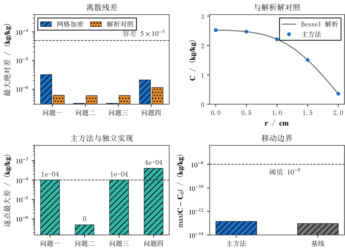
图 12 数值可信度的四类证据
