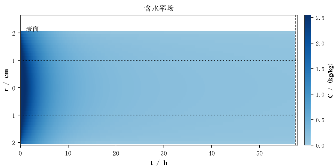
图 10 问题三含水率场（附录图）
