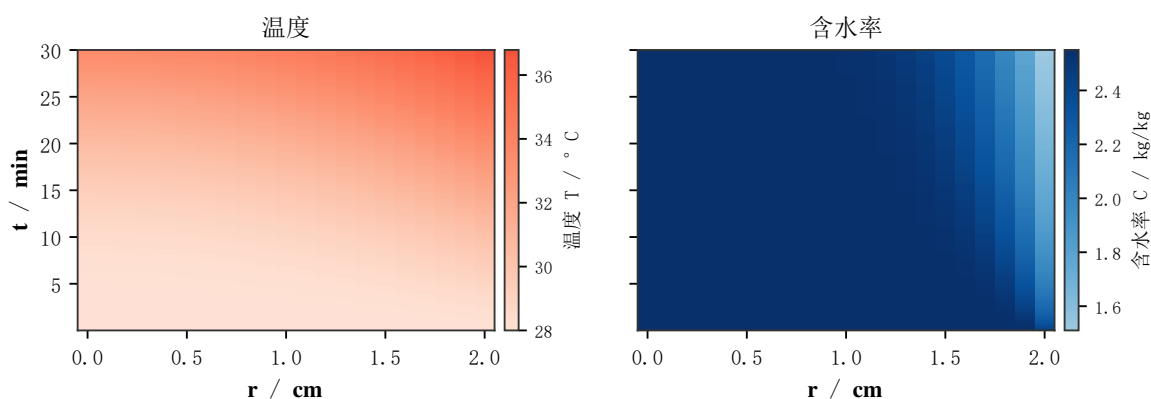
图 6 预热阶段温湿场（附录图）
