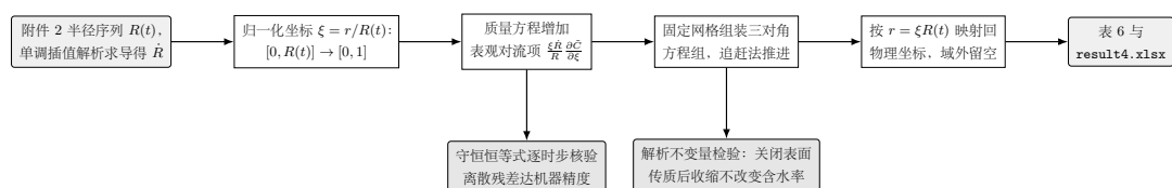
图 11 问题四的求解流程。由附件 2 求出半径及其变化率，经归一化坐标把移动域映射为固定域，在固定网格上叠加表观对流项后逐时步推进，最后映射回物理坐标输出。
