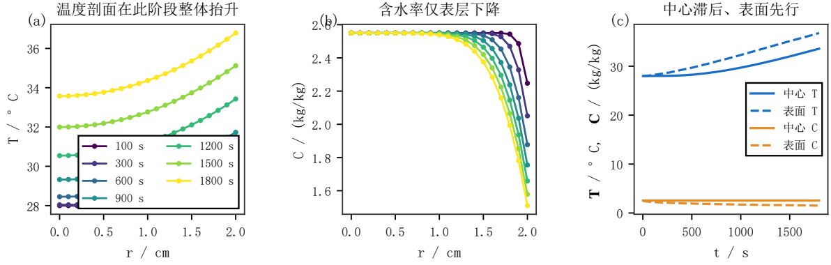
图 5 预热平衡阶段 (0 ~ 1800 s) 的温度与水分场。(a)、(b) 为七个报告时刻的径向剖面；(c) 为中心与表面时程。1800 s 时中心温度 33.5753 °C、表面 36.7856 °C；干基含水率中心仍为 2.55 kg/kg，仅表面降至 1.5102 kg/kg。
