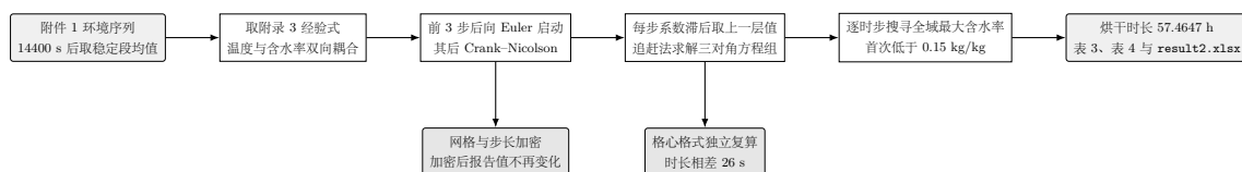
图 7 问题二的求解流程。与问题一的差别在于物性改为温度与含水率双向耦合的经验式，时间推进需以三步后向 Euler 启动，以抑制环境跃变引起的振荡。
