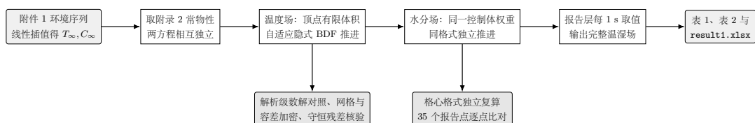
图 4 问题一的求解流程。温度场与水分场因物性为常数而相互独立，可分别推进；两场共用同一套控制体权重与界面系数。
