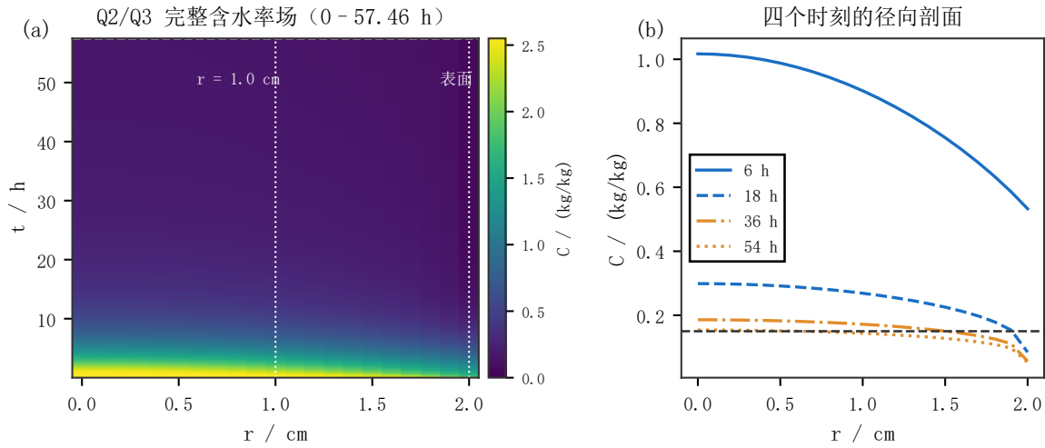
图 10 问题三完整含水率场 (0 ~ 57.46 h, 附录图)。(a) 径向-时间分布，虚线标出烘干结束时刻；(b) 四个时刻的径向剖面。
