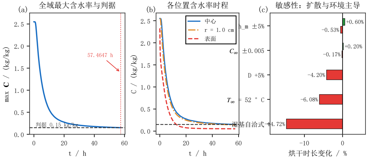
图 8 长时程烘干过程与敏感性。(a) 全域最大干基含水率随时间的演化与 0.15 kg/kg 判据，判据于 57.4647 h 首次越过；(b) 三个位置的含水率时程；(c) 单项扰动对烘干时长的影响。
