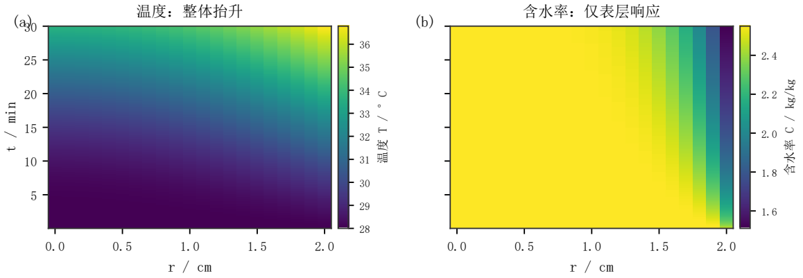
图 6 预热阶段温湿场的完整时空分布（附录图）。左：温度；右：干基含水率。
