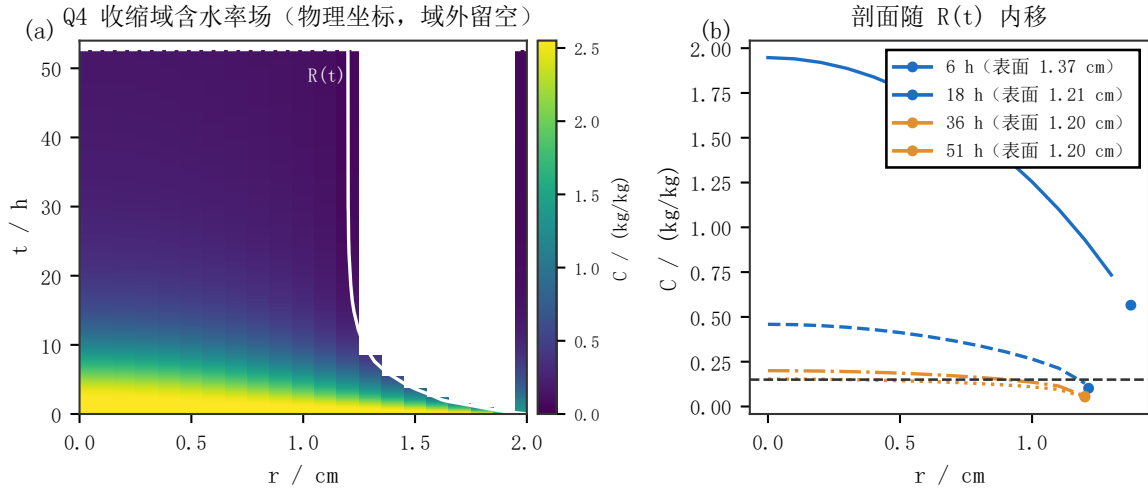
图 13 问题四收缩域内的含水率场（附录图，物理坐标）。(a) 径向-时间分布，白线为 R(t) ，域外留空；(b) 四个时刻的径向剖面，圆点为该时刻的表面位置。
