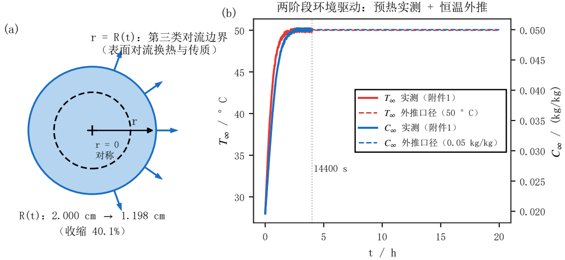
图 3 模型几何与边界驱动。(a) 药材按一维径向轴对称处理， r = 0 处对称、 r = R(t) 处第三类对流；(b) 预热阶段的环境温湿度取附件 1 实测序列（线性插值），14400 s 之后取稳定段实测均值，维持 T_\infty = 50^\circ\text{C} 、 C_\infty = 0.05 \text{ kg/kg} 。该外推为模型设定，并非实测数据。
