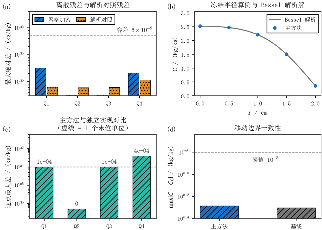
图 14 数值可信度的四类证据。(a) 网格加密残差与解析解对照残差；(b) 问题四的固定半径算例与 Bessel 级数解析解的对照；(c) 本文方法与独立实现的逐点最大差，虚线为一个末位单位对应的容差；(d) 问题四关闭表面传质后干基含水率的偏移量与其阈值。
