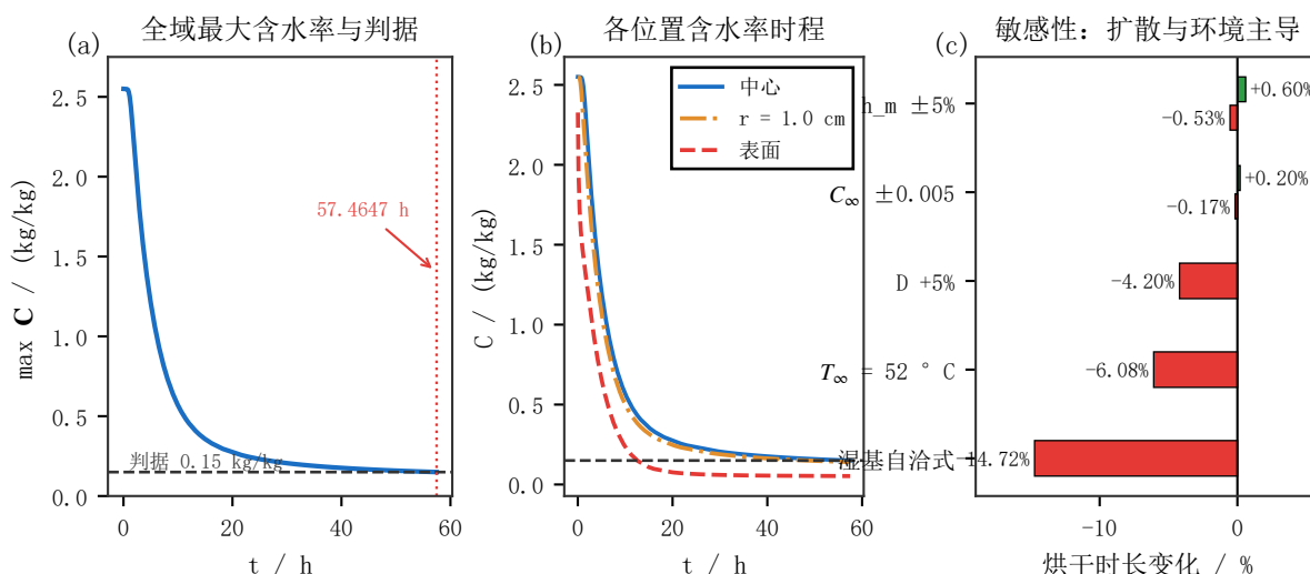
图 6 长时程烘干过程与敏感性。(a) 全域最大干基含水率随时间的演化与 0.15 kg/kg 判据；在题目给定的 h_m 、附录 3 经验式与恒温段环境口径下，判据于 57.4647 h 首次越过。(b) 三个位置的含水率时程。(c) 单项扰动对烘干时长的影响。
