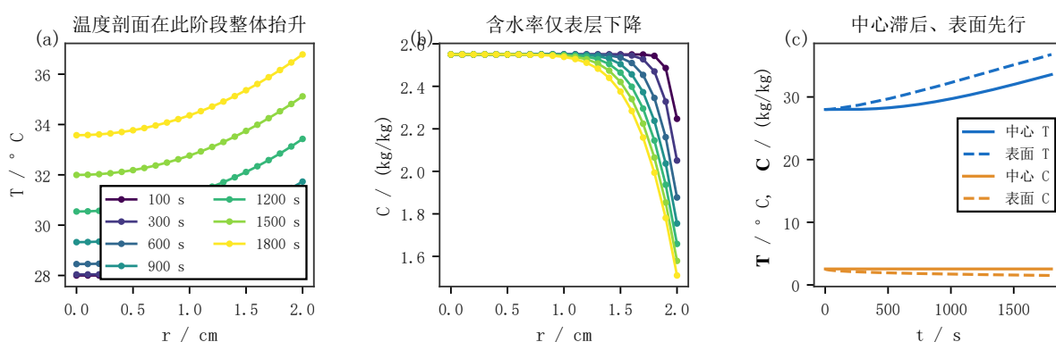
图 4 预热平衡阶段 ( 0 \sim 1800 s) 的温度与水分场。(a)、(b) 为七个报告时刻的径向剖面；(c) 为中心与表面时程。在题目给定的 h_m 与附录 2 经验式下，1800 s 时中心温度 33.5753^{\circ}\text{C} 、表面 36.7856^{\circ}\text{C} ；干基含水率中心仍为 2.55 \text{ kg/kg} ，仅表面降至 1.5102 \text{ kg/kg} 。
