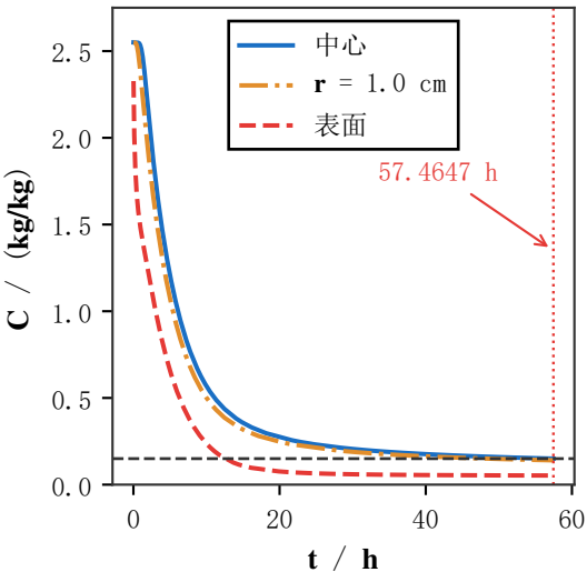
含水率时程
