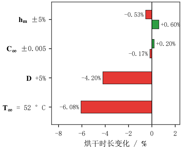
敏感性
