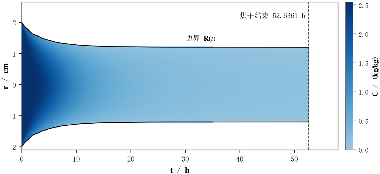
收缩域含水率场
