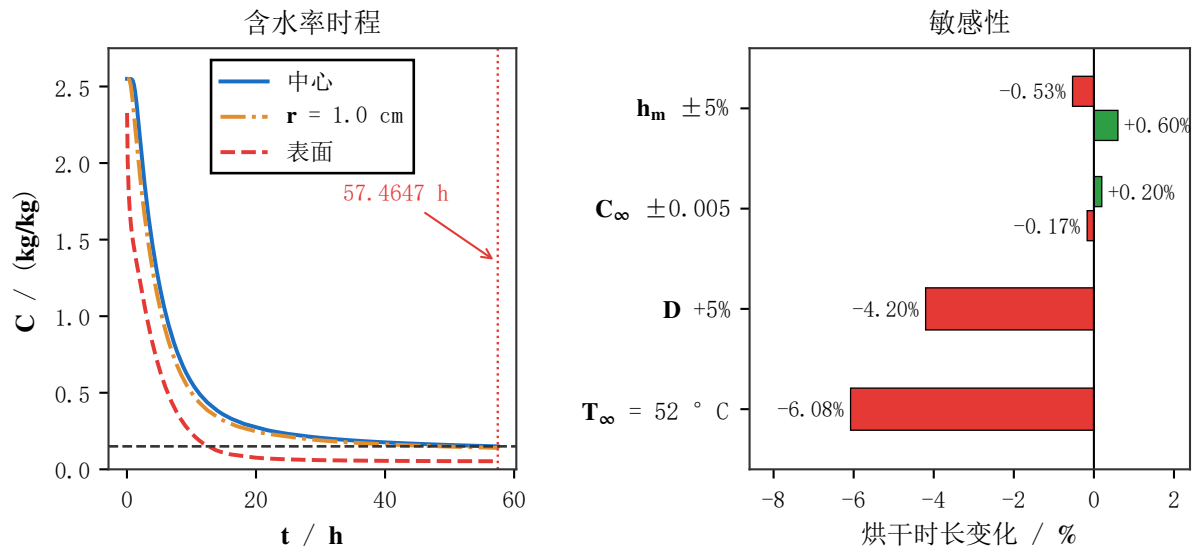
图 9 长时程烘干与敏感性
