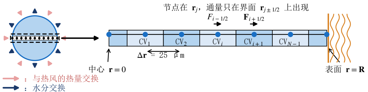
图 2 顶点型有限体积离散示意
