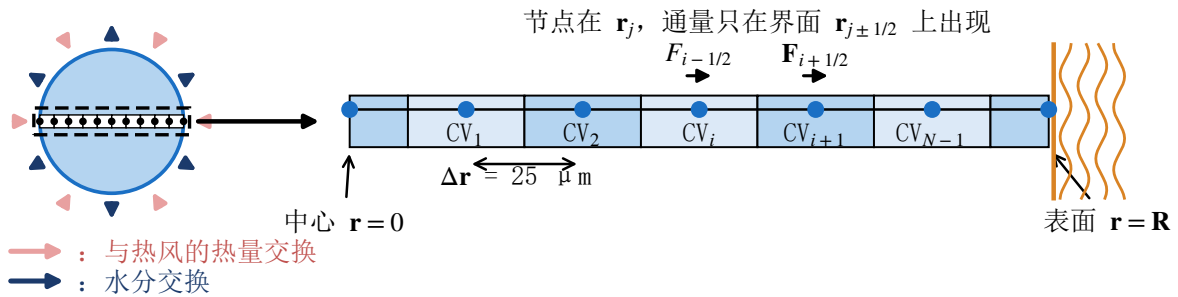
图 4 顶点型有限体积离散示意
