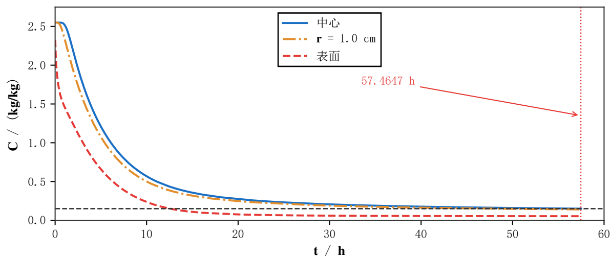
图 9 三个位置的含水率时程
