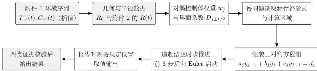
图 3 统一求解流程。由环境序列与几何数据出发，经控制体权重与界面系数构造，按问题选取物性经验式与时间格式，最后由追赶法逐时步推进并输出报告值。
