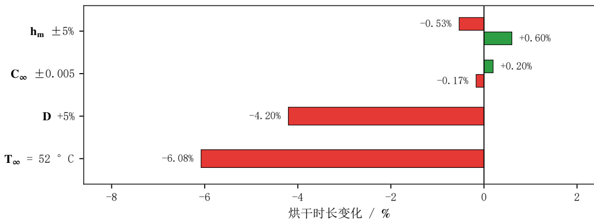
图 11 烘干时长对单项扰动的响应（问题二与问题三）
