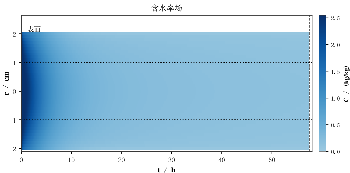
图 10 问题三含水率场（附录图）
