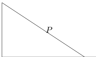
Figura 1.1 — O gráfico de uma função linear.
