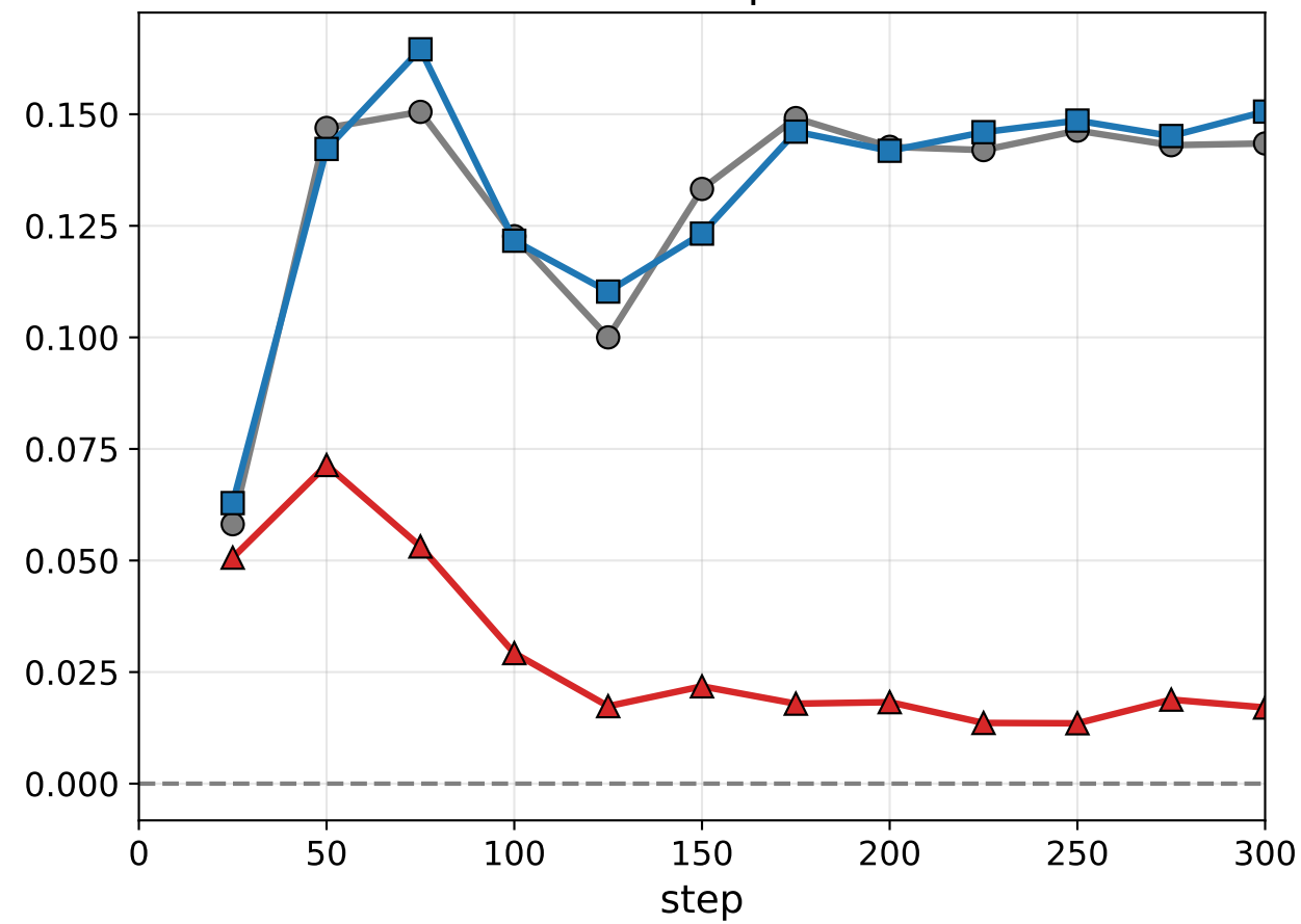
triviaqa
