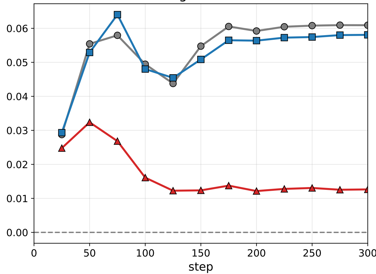
gsm8k
