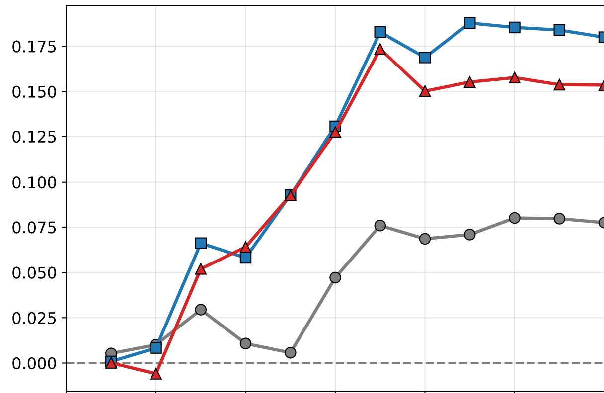
triviaqa
