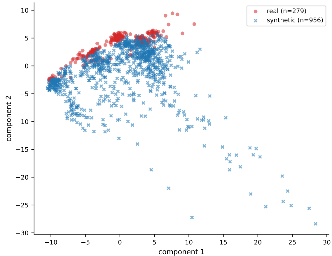
PCA (2 components)
