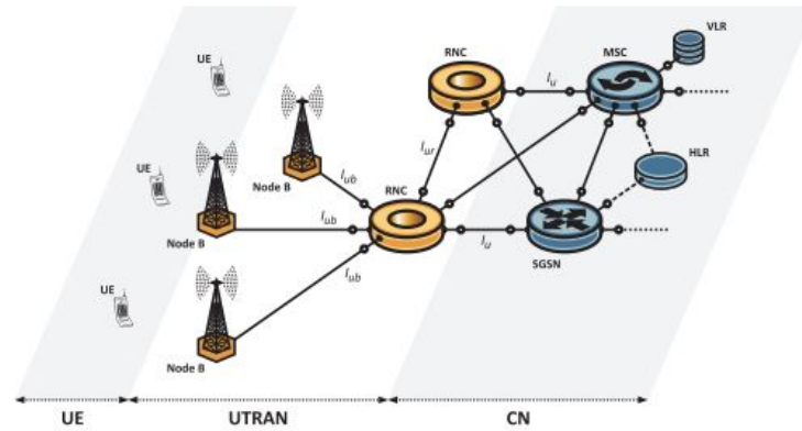
Arquitectura de la Red 3G
