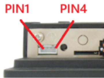
FAN Connectors
