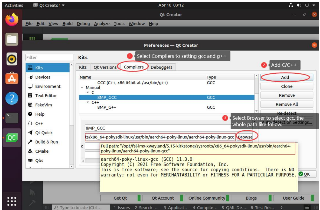
Compilers -gcc
