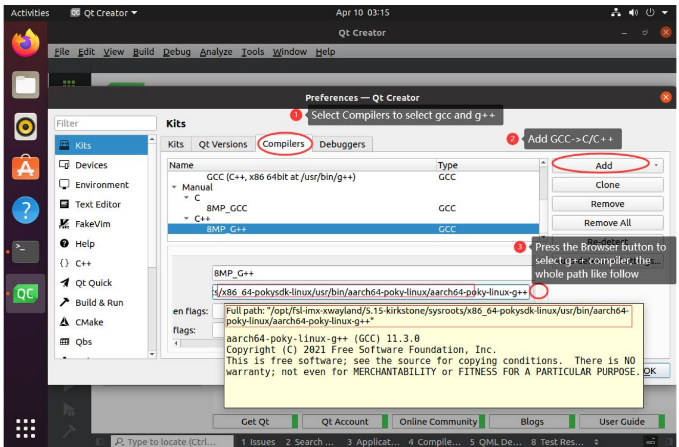
Compilers -g++
