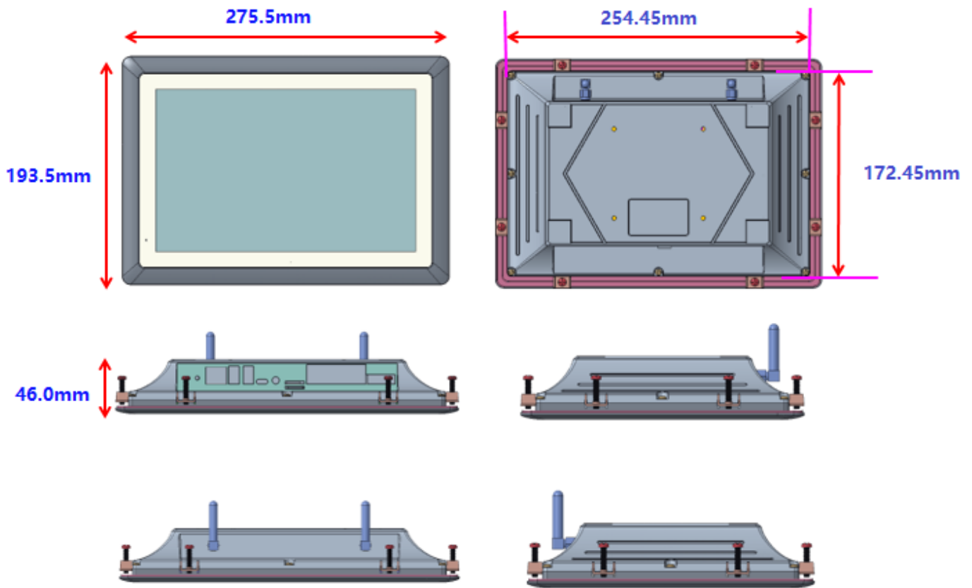
Dimensions (PPC-A35-101)
