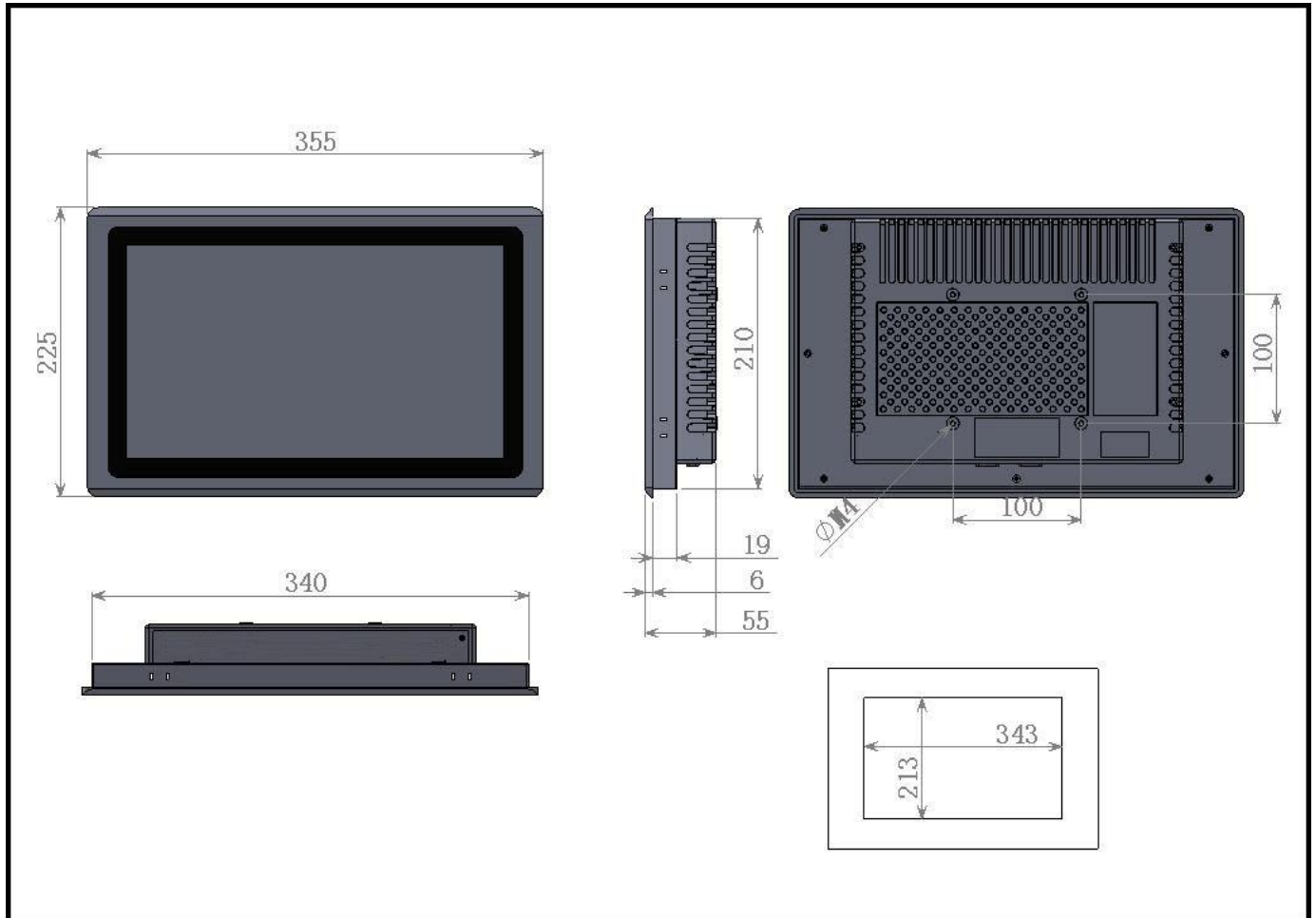
Dimensions (PPC-A35-133)
