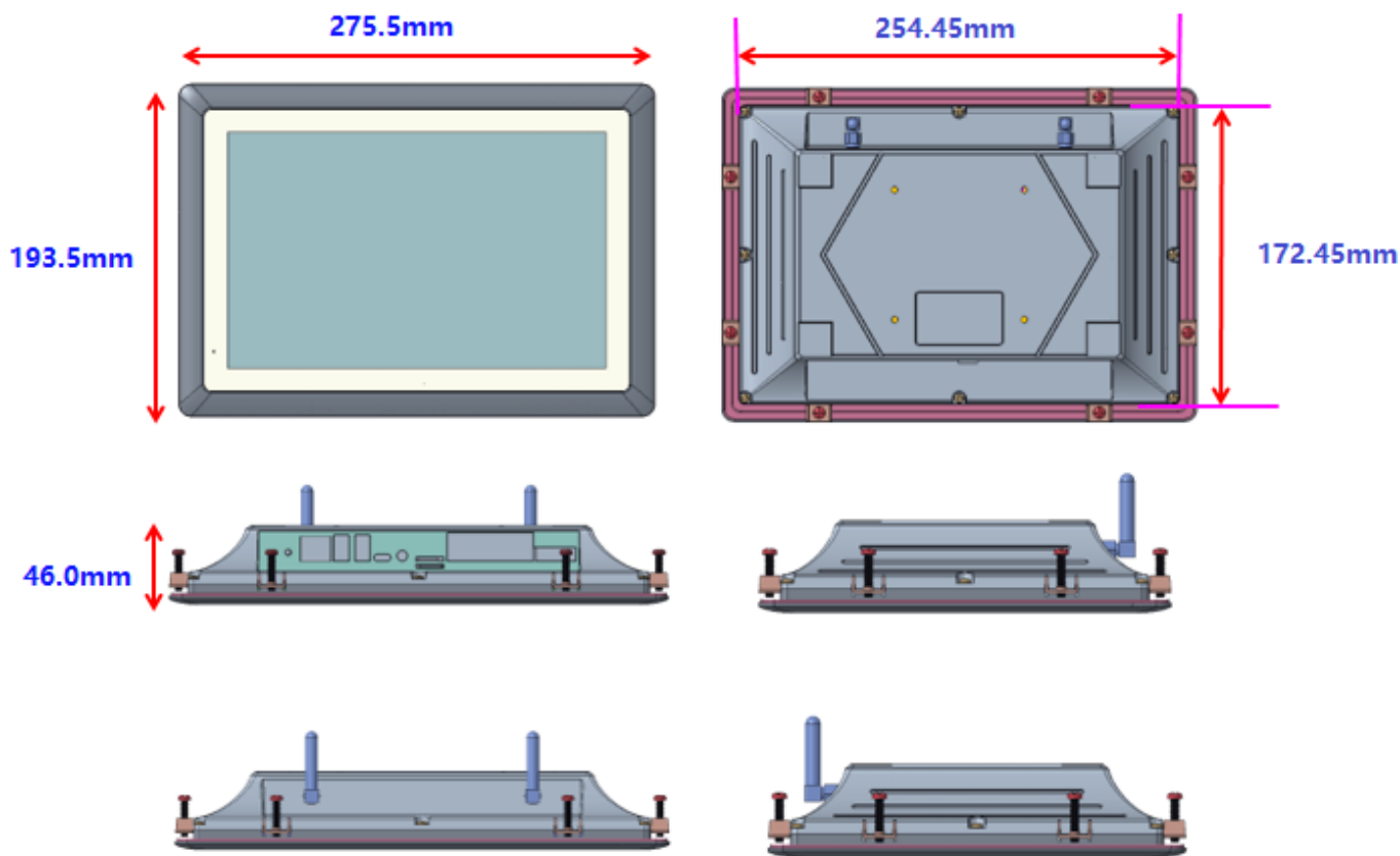
Dimensions (PPC-A35-101)
