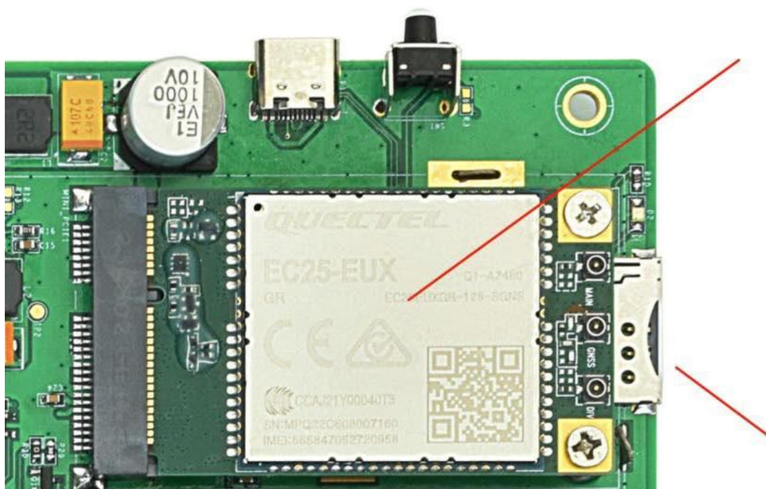
3G/4G/LTE Module
